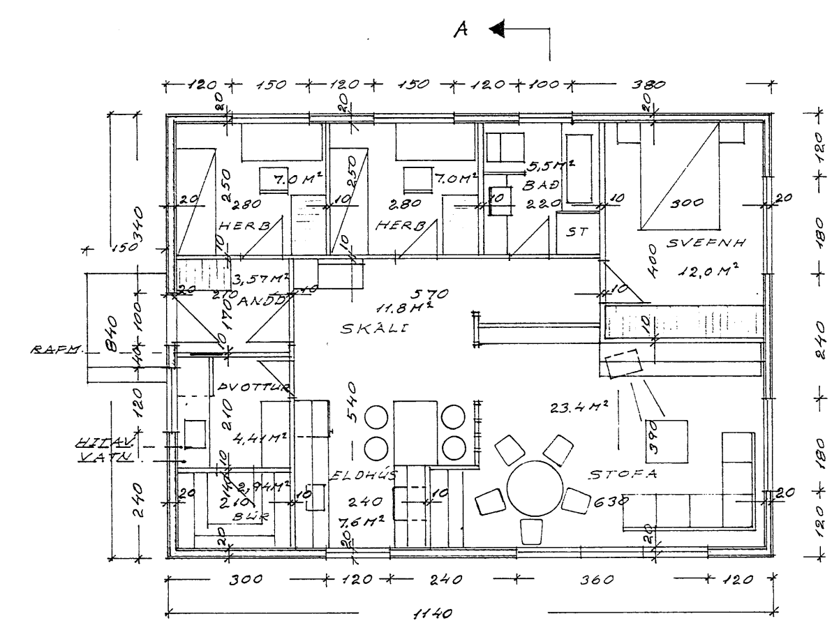
GRUNNMYND 1:100
