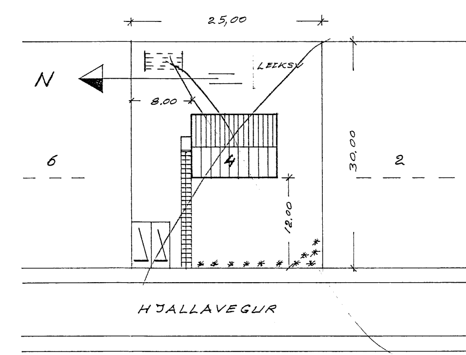
AFSTAÐA 1:500
