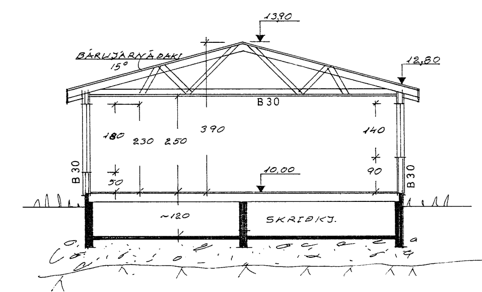
SNID A-A 1:100
