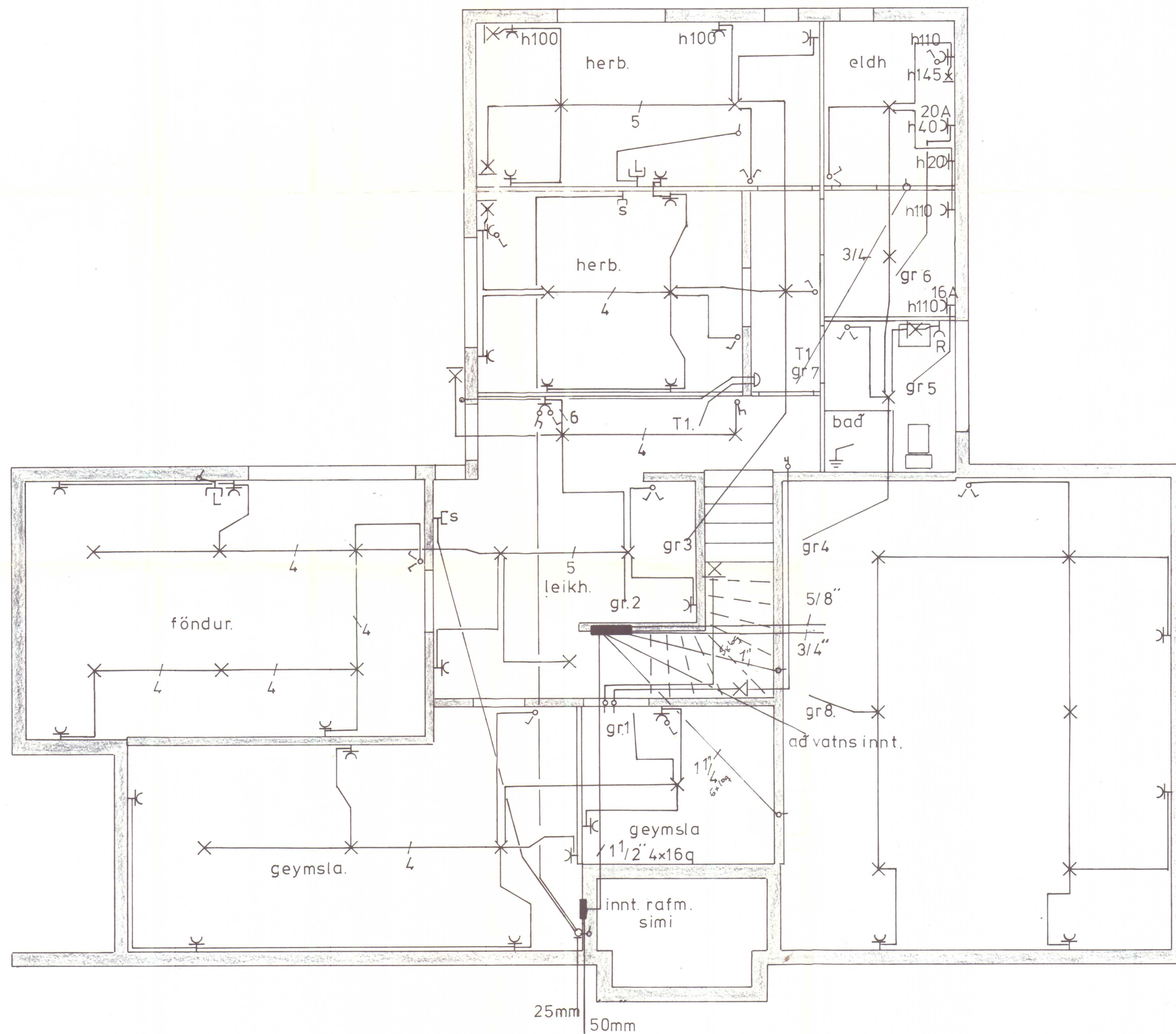
grunnmynd neðrihæð
