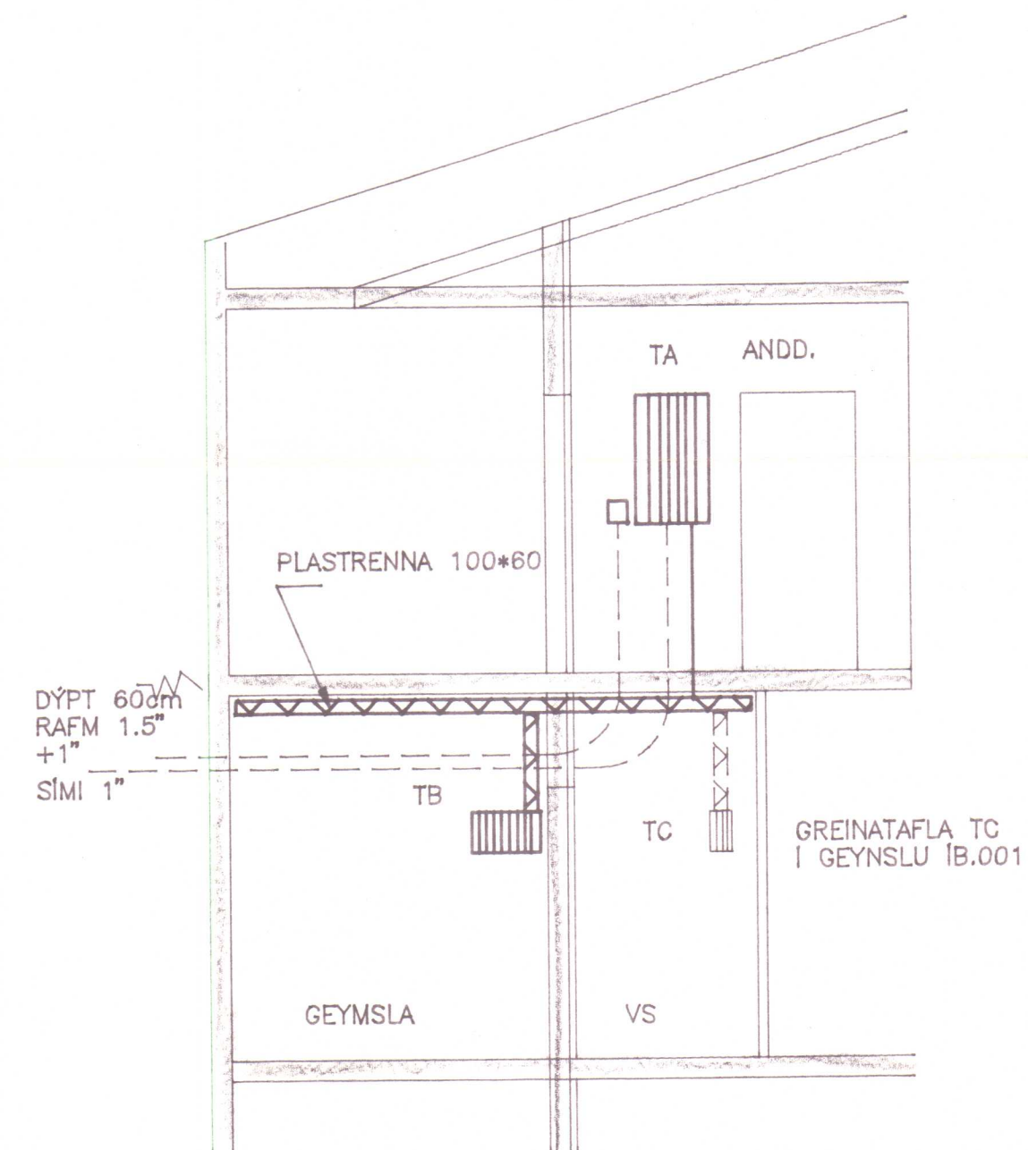
SNÍÐ A-A 1:50
