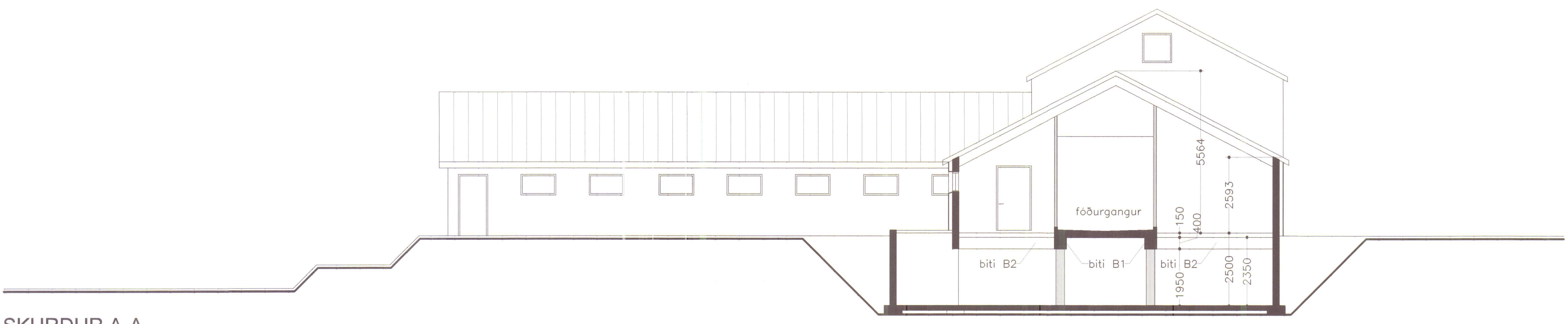
SKURÐUR A-A
