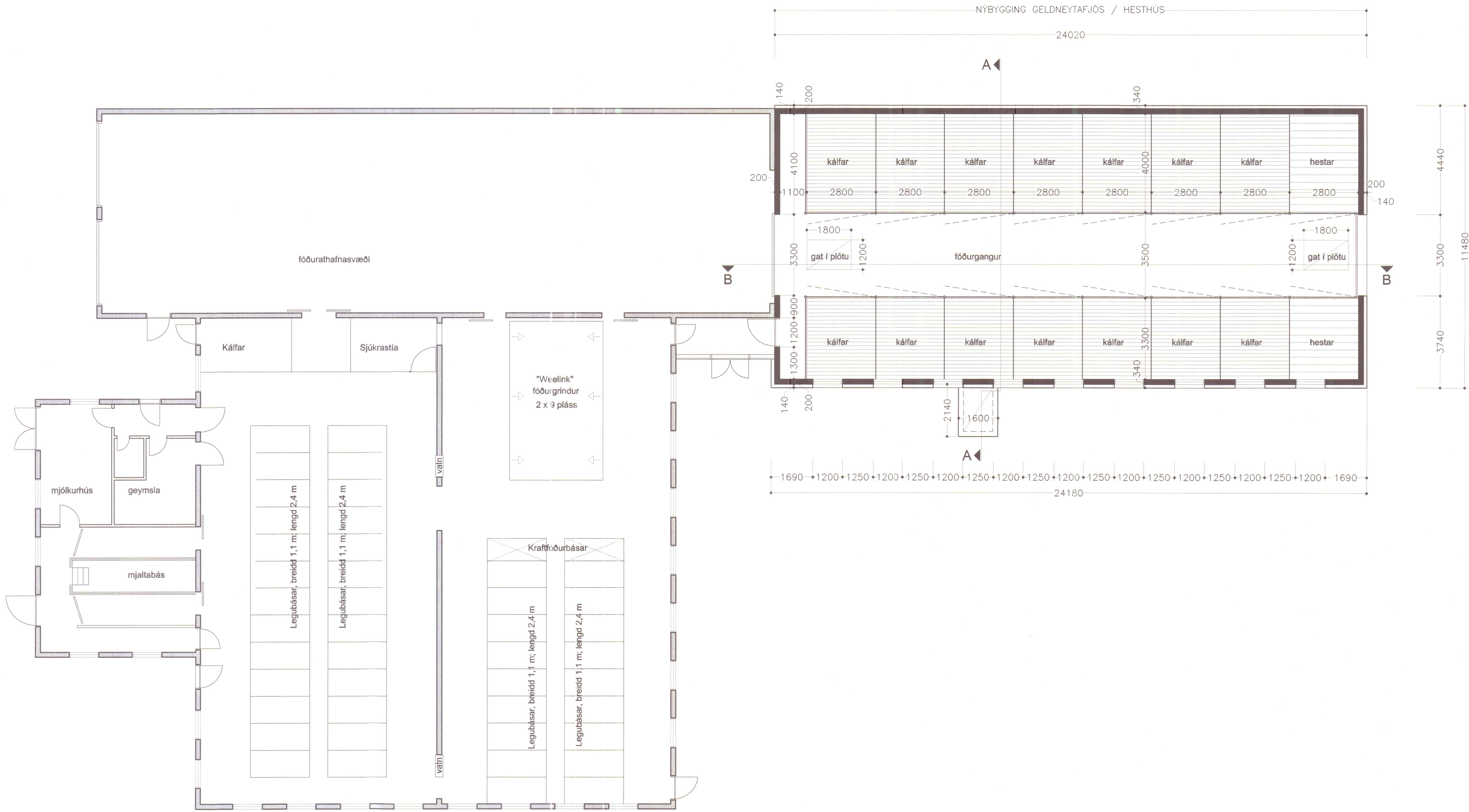
GRUNNMYND 1:100
