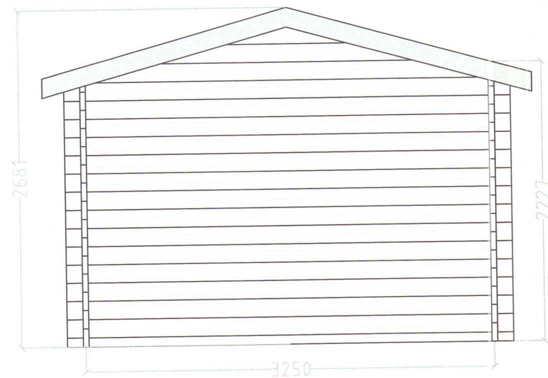
Snið C-C
