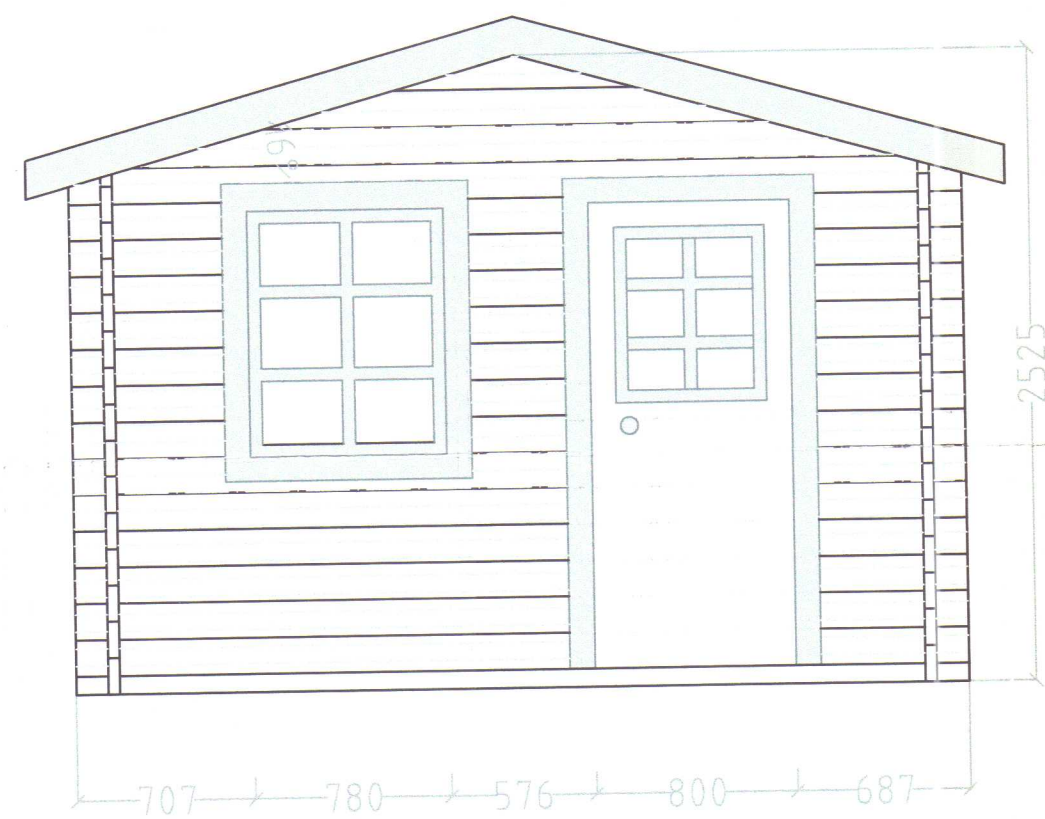
Snið A-A
