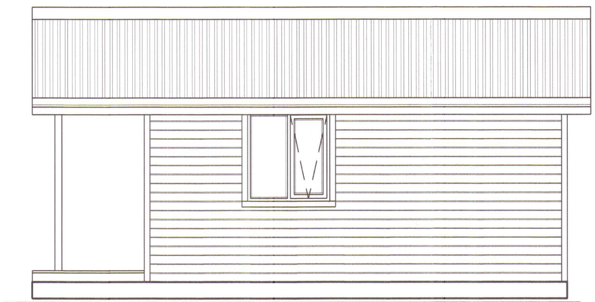
○ Norðurhlið - 1:50
