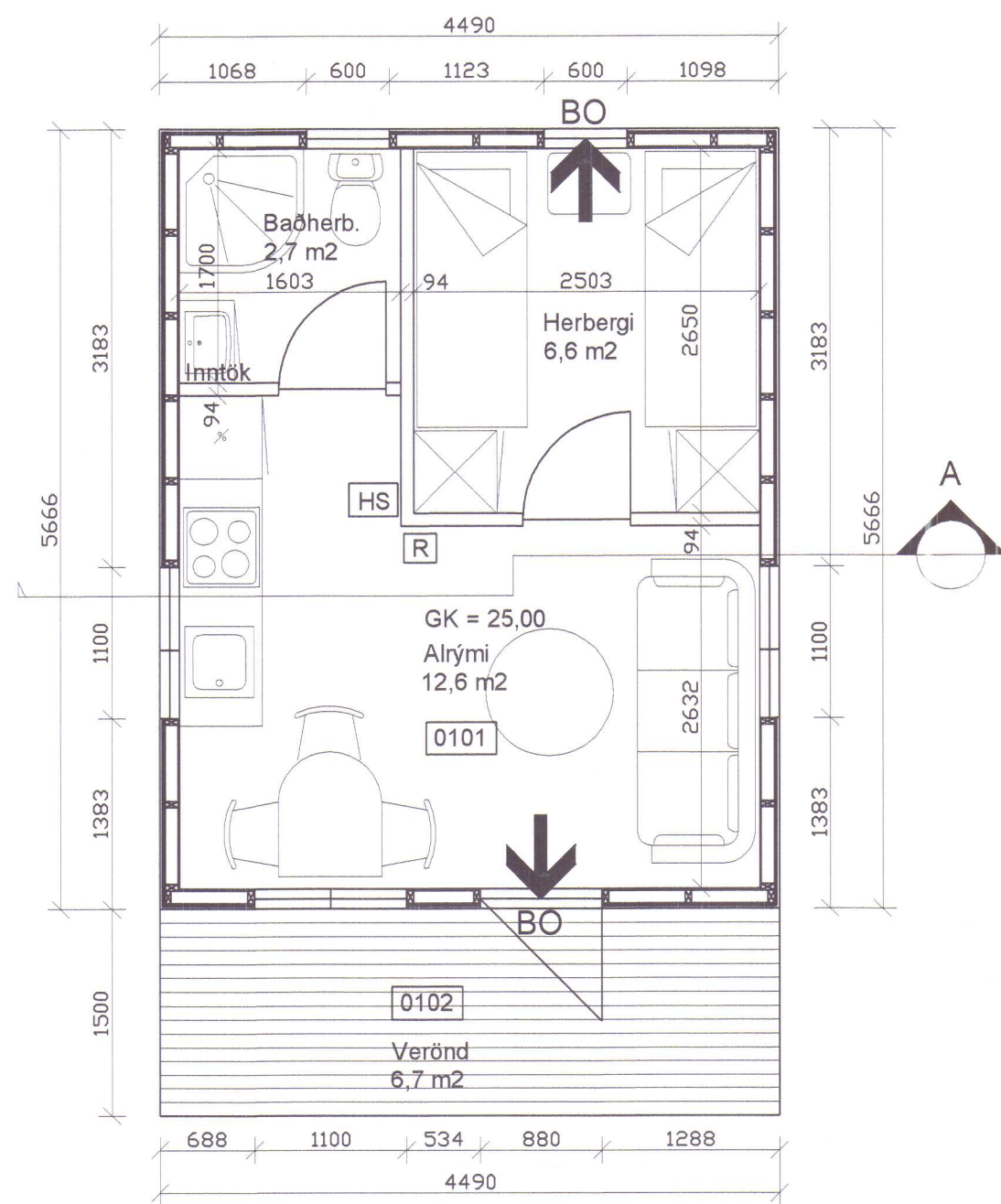
○ Grunnmynd - 1:50
