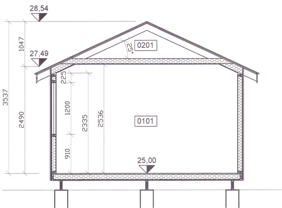
○ Snið A - 1:50
