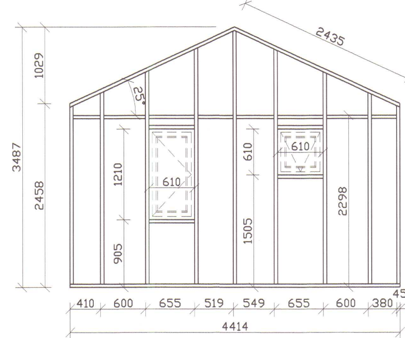
V3 ÚTLIT - 1:50
