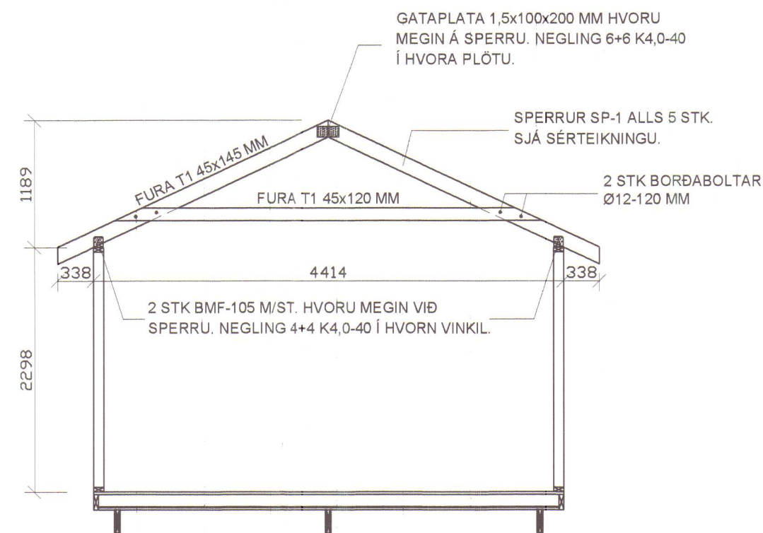
SNÍÐ 5 - 1:50
