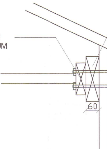
DEILI 4 - 1:10
