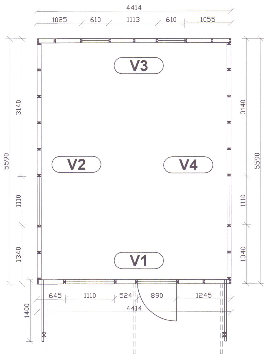
GRUNNMYND - 1:50
