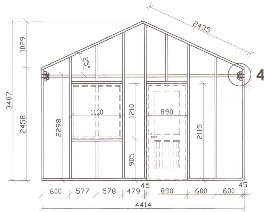
V1 ÚTLIT - 1:50
