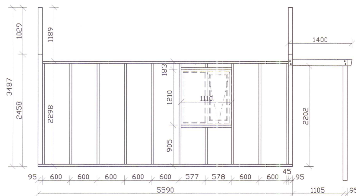
V2 ÚTLIT - 1:50
