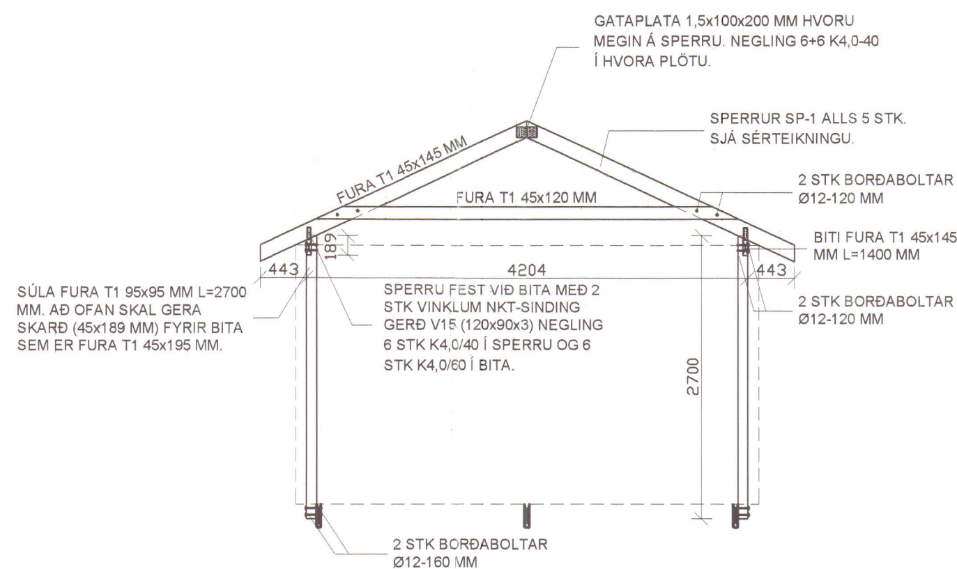
SNÍÐ 6 - 1:50
