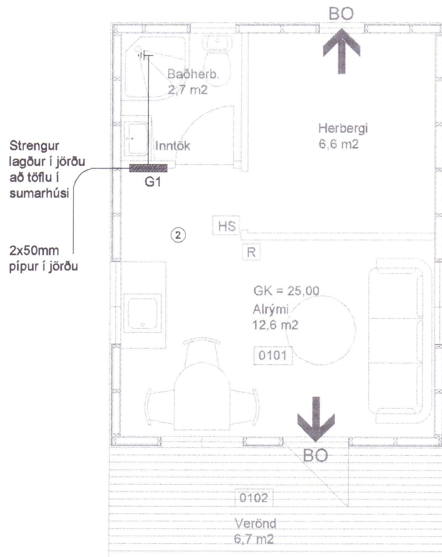
GRUNNMYND 1:50
