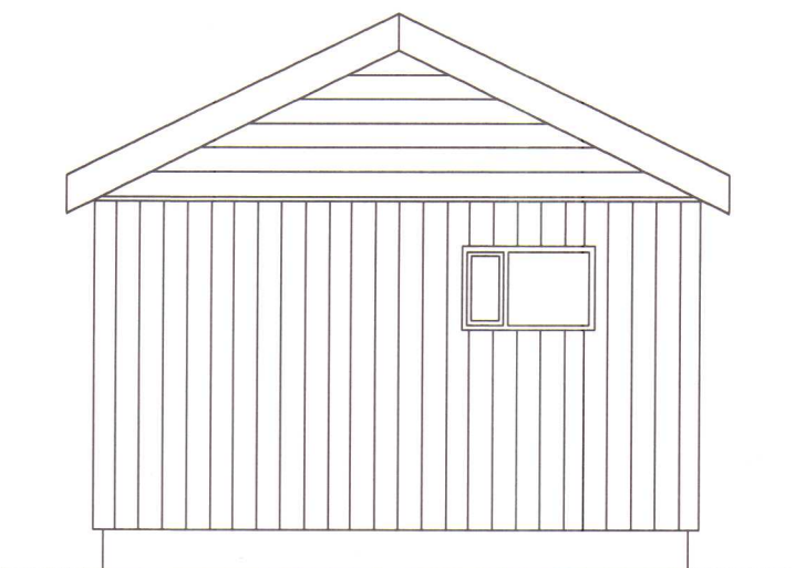
Útlit, Austur 1:50
