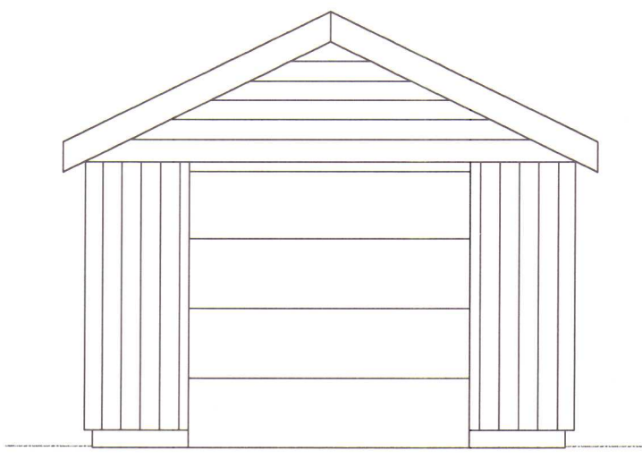
Útlit, Vestur 1:50
