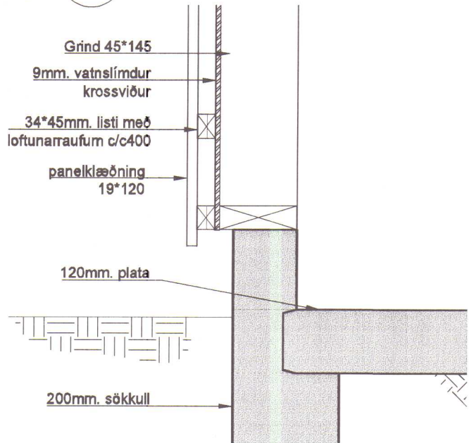
Deili 1:10
