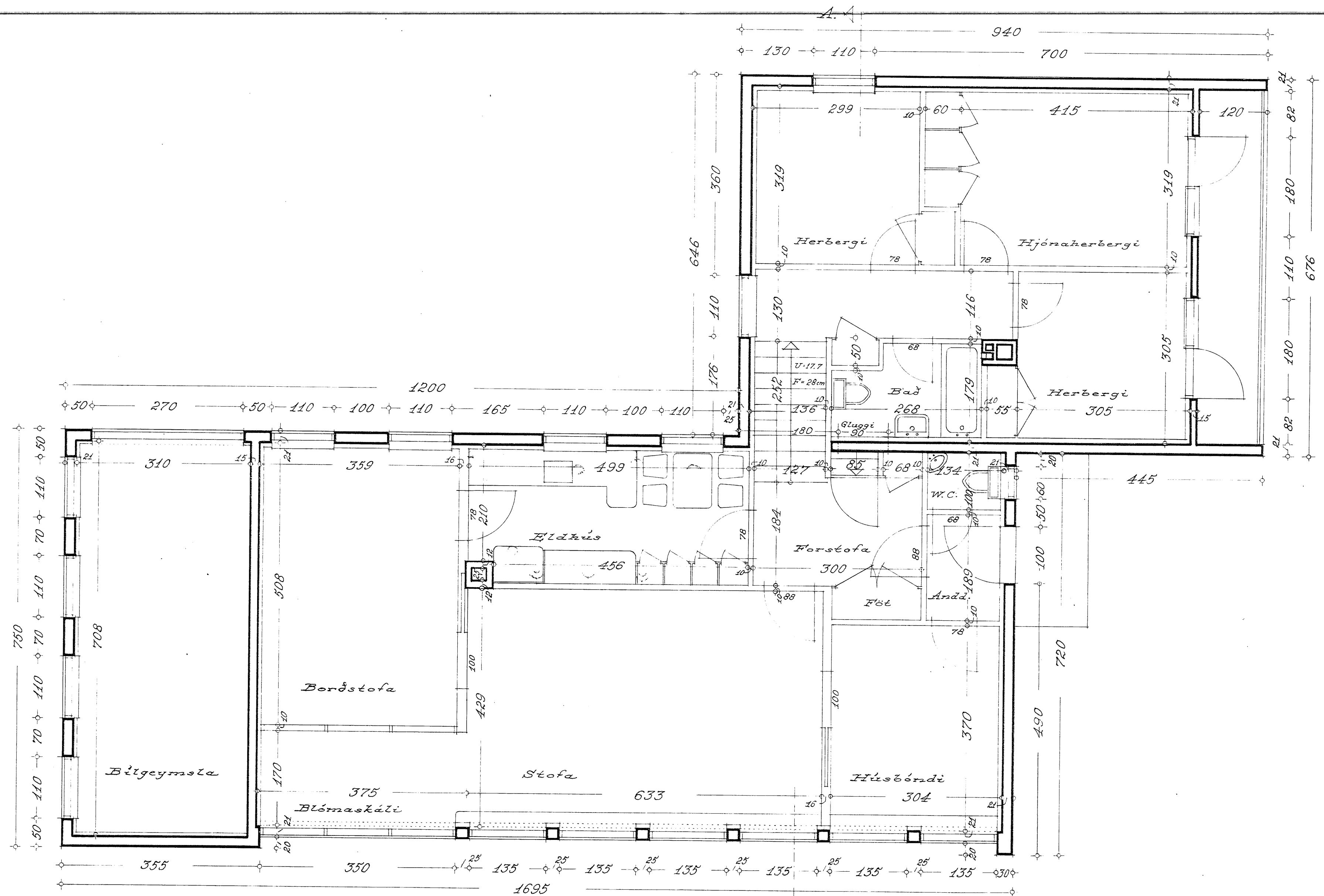
Grunnmynd 1. hæðar
