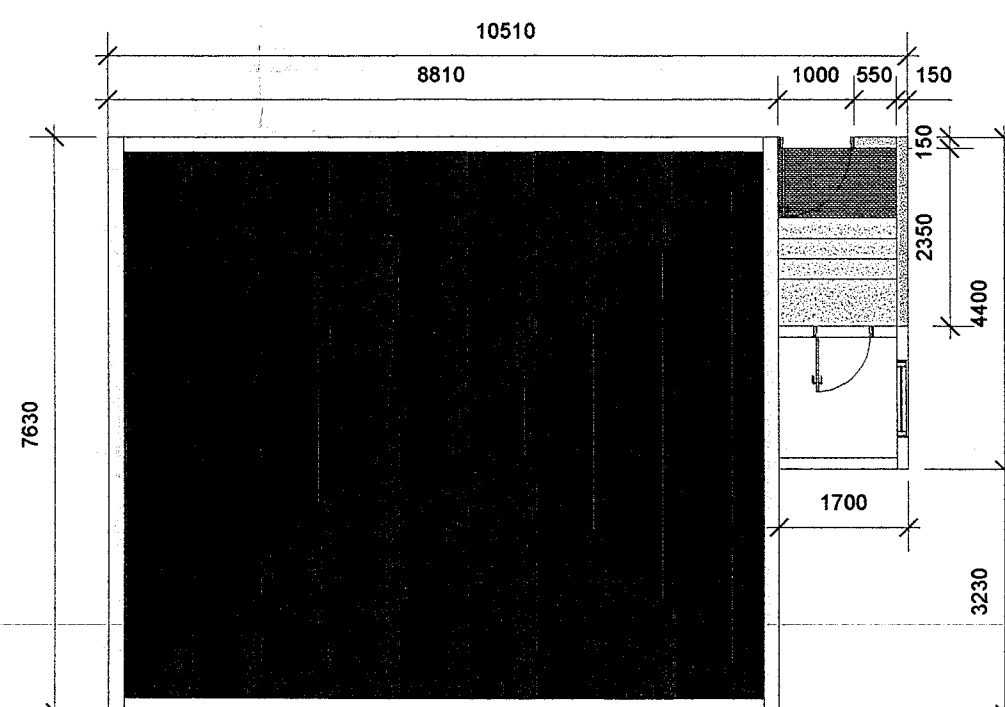
GRUNNMYND / ÞAKMYND 1:100
