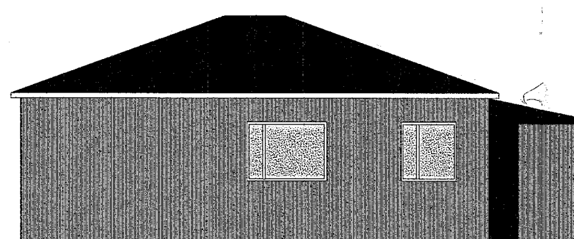
ÚTLIT AUSTUR. 1:100
