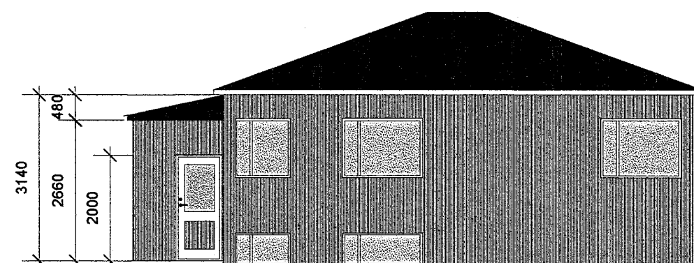
ÚTLIT VESTUR 1:100
