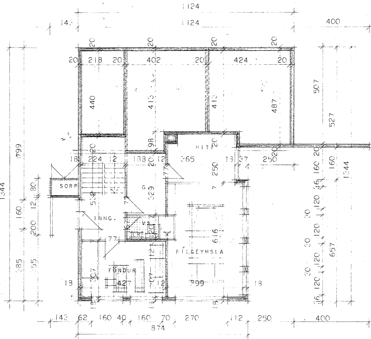
GRUNNMYND KJALLARA
