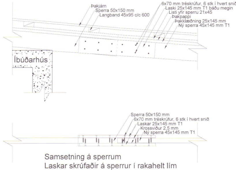
Hlutateikning B-1 Mkv. 1:20
