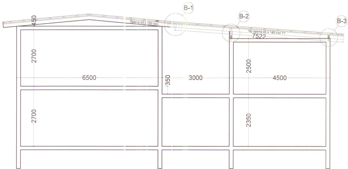
BURÐARVIRKI - SNIÐ MKV. 1:100
