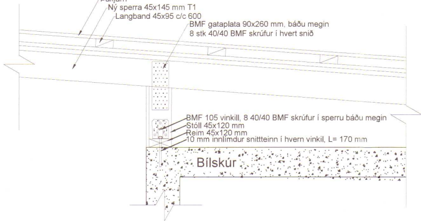
Hlutateikning B-2 Mkv. 1:20
