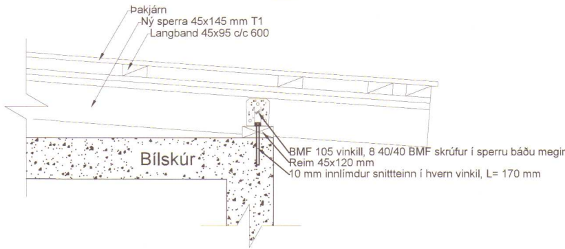
Hlutateikning B-3 Mkv. 1:20
