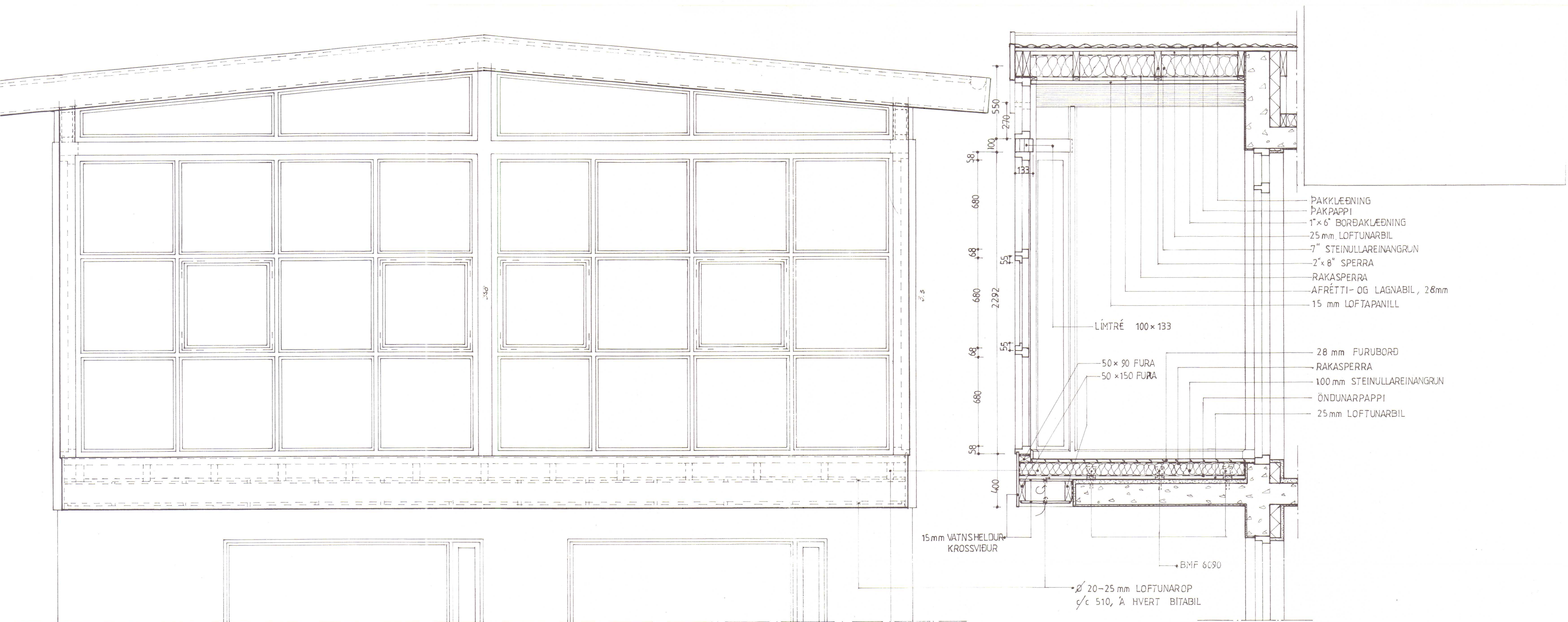
ÚTLIT MÓT VESTRI 1:20
