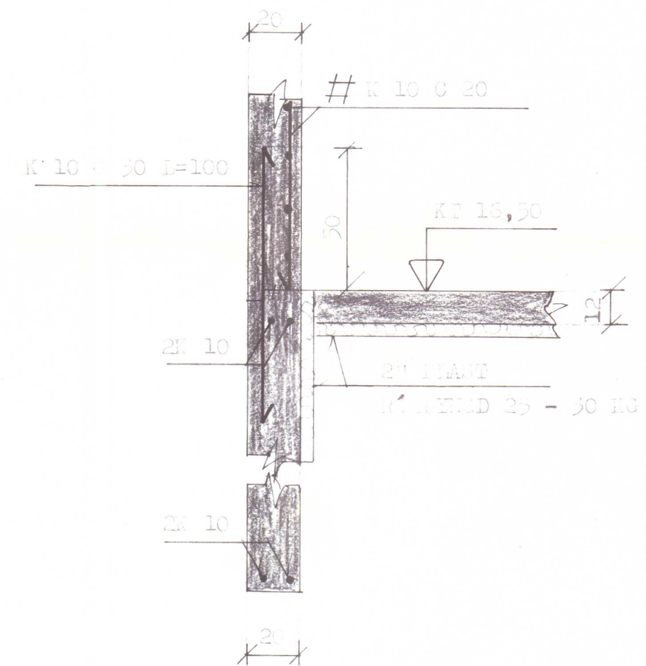
SNID D - D. 1:20.
