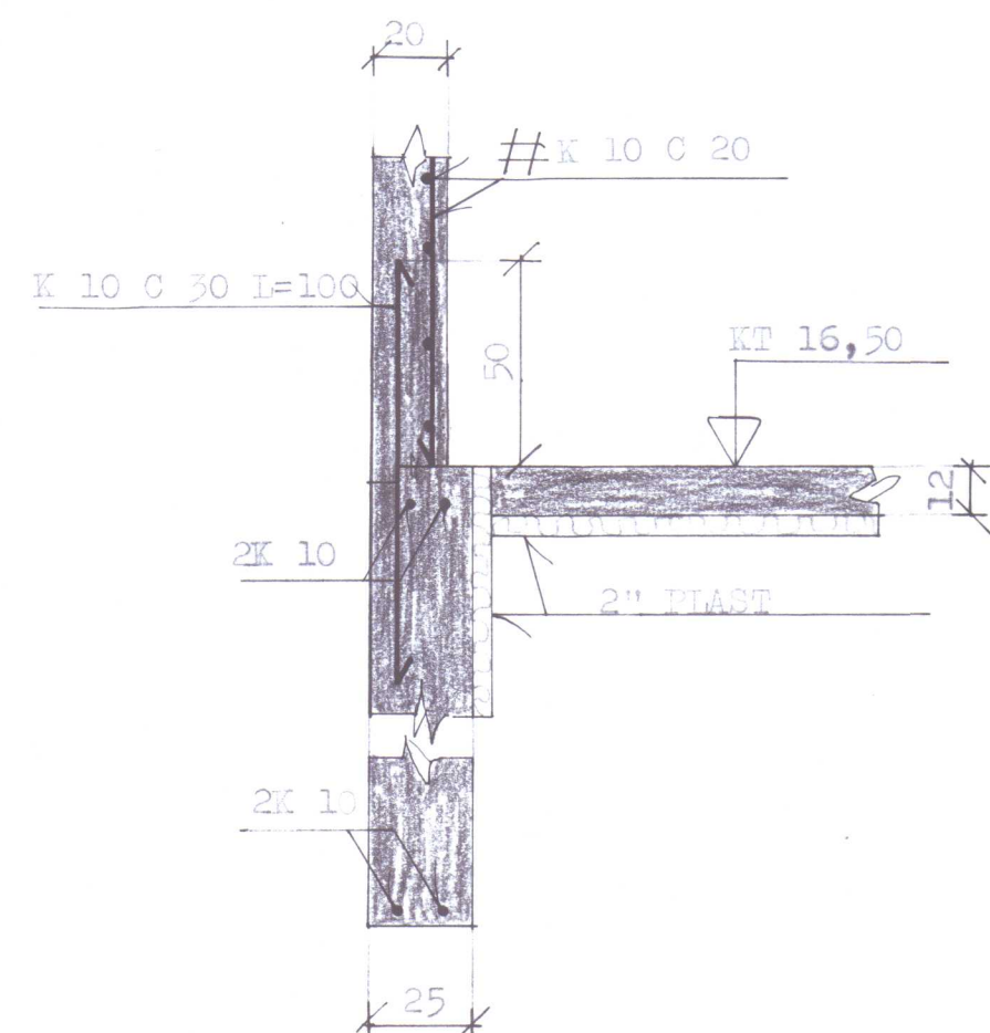
SNID E - E. 1:20.
