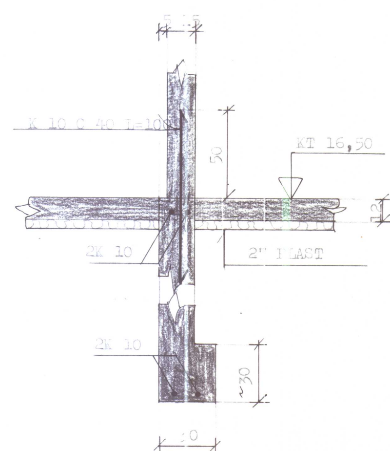
SNID F - F. 1:20.
