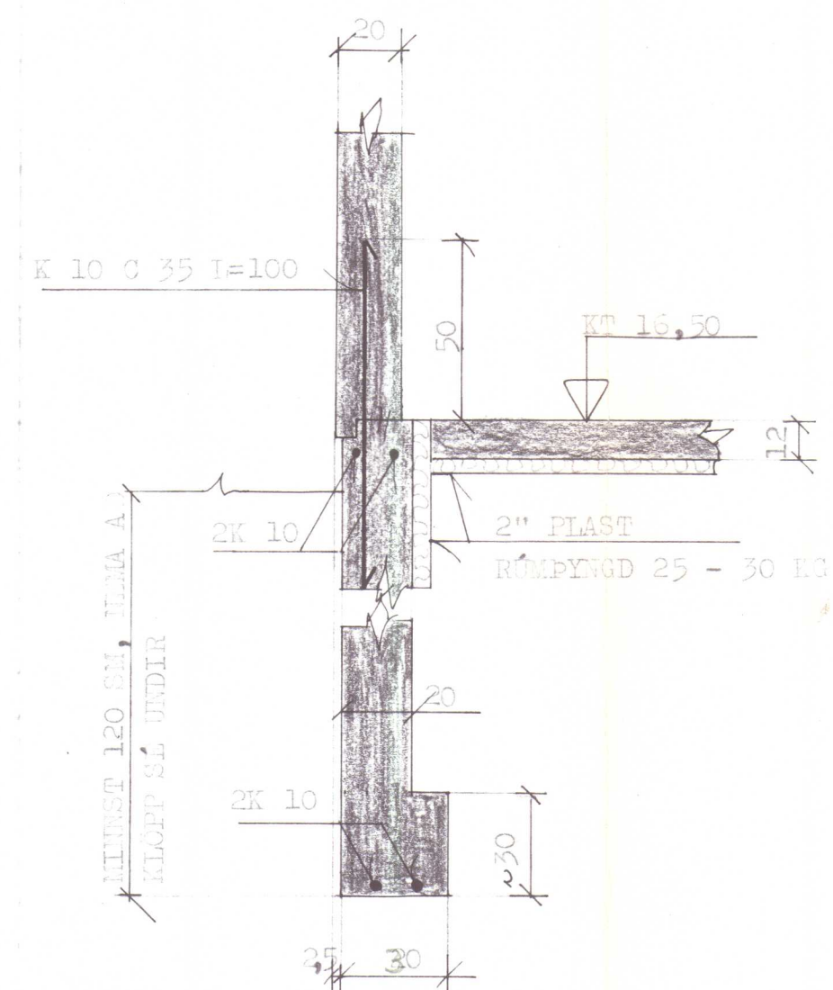
SNID A - A. 1:20.
