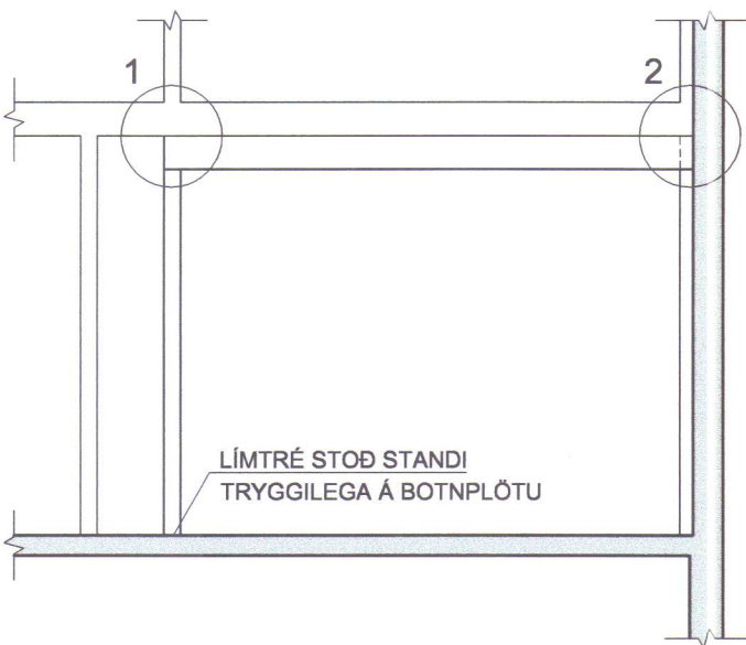
SNID A mkv. 1:50
