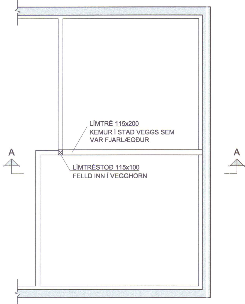
GRUNNMYND mkv. 1:50
