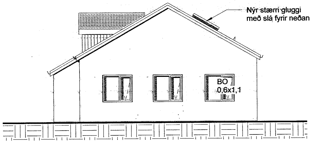
1 SUÐURGAFL 1:100
