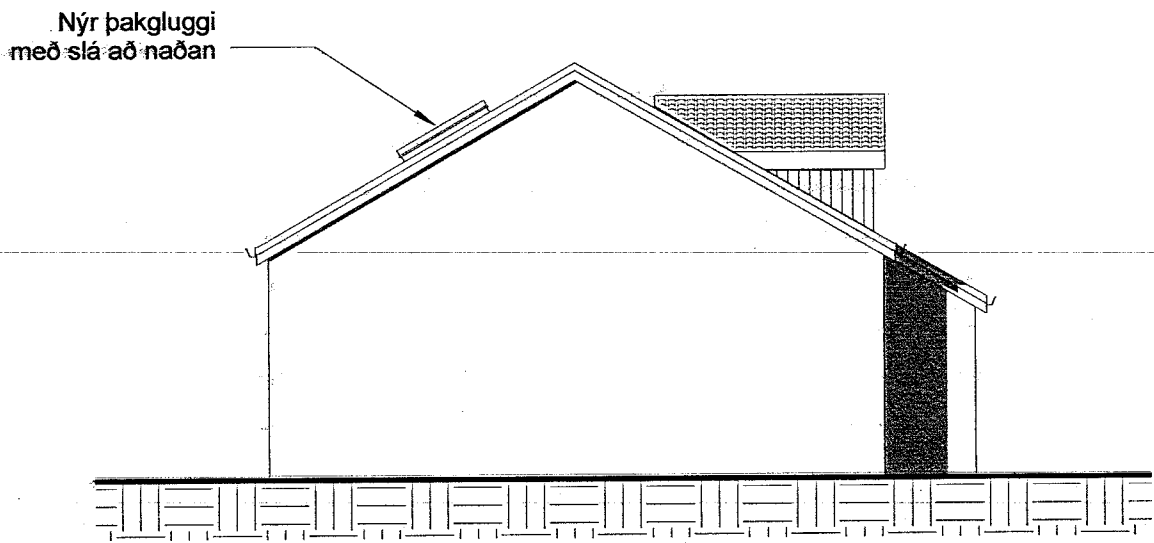
4 NORÐURGAFL 1:100
