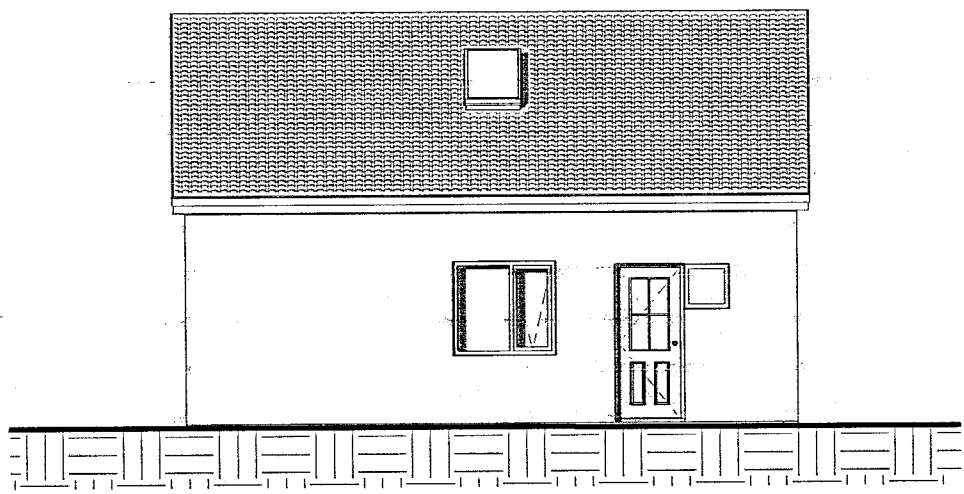
2 AUSTURHLIÐ 1:100
