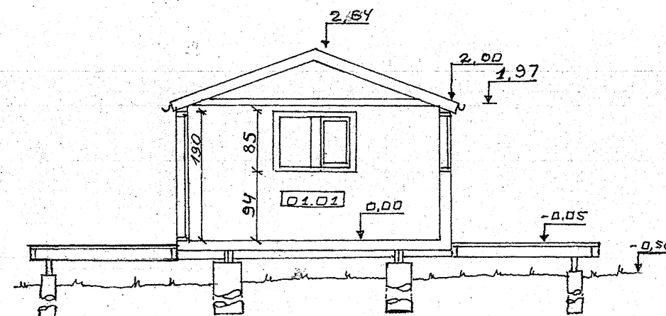
SNÍÐ A-A M 1:50
