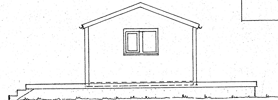
SÚÐURHLÍÐ M 1:50
