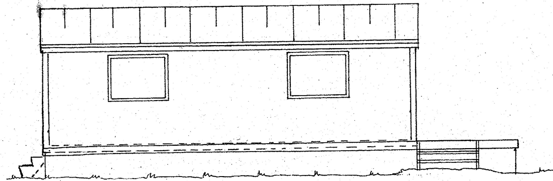
VESTURHLÍÐ M 1:50
