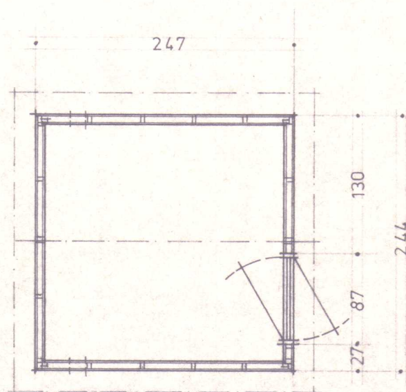
GRUNNMYND
