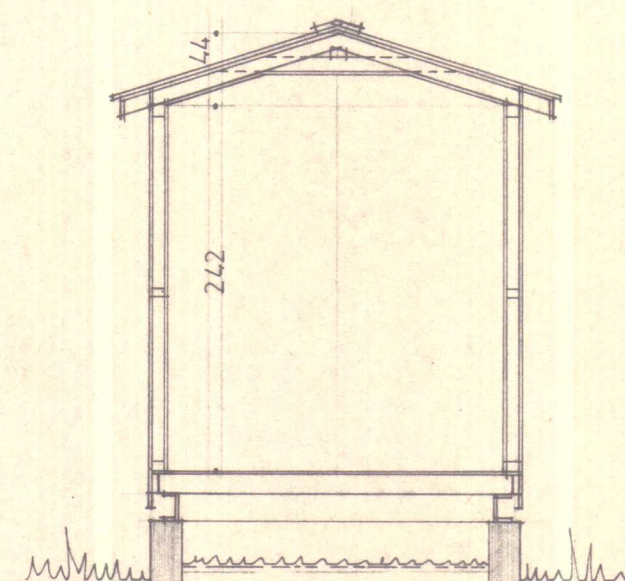
SNIÐ
