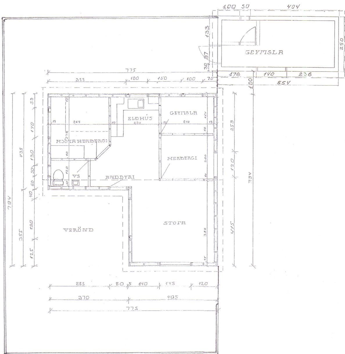
GRUNNFLÝND 1:100
