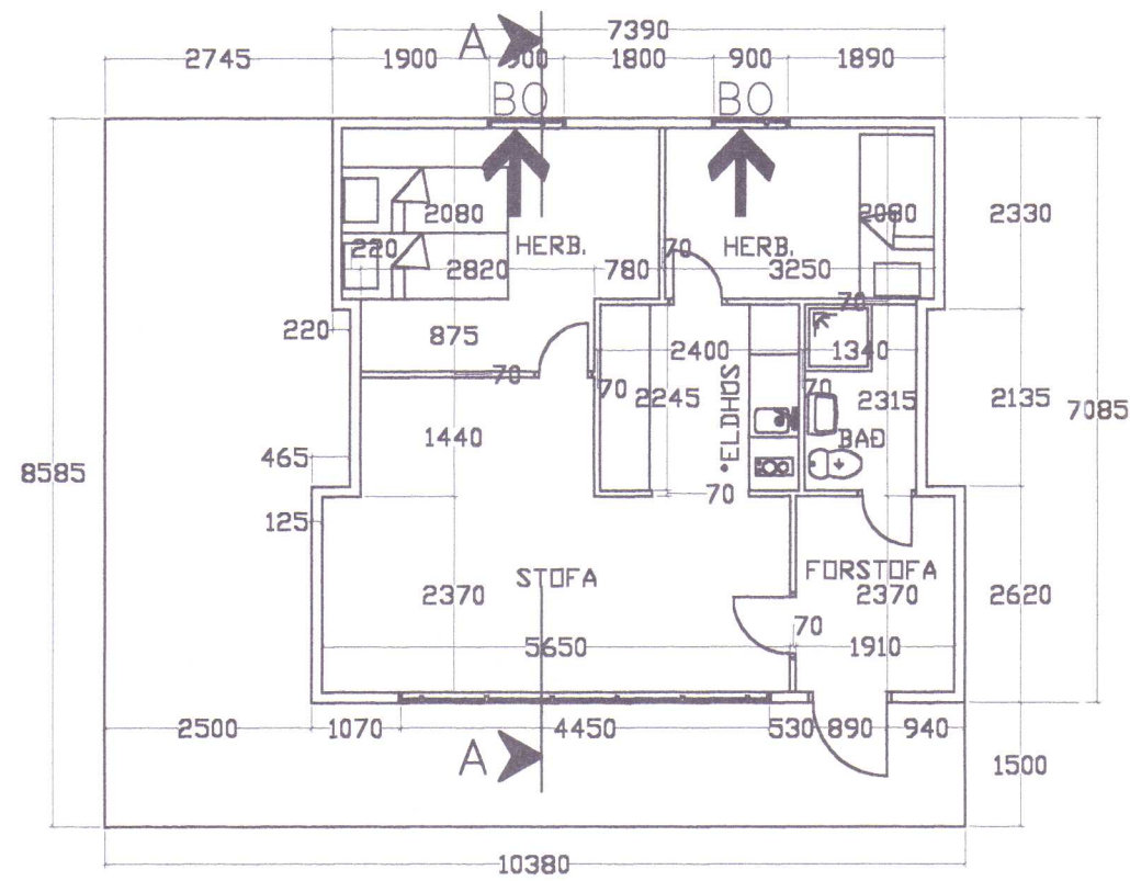
GRUNNMYND
