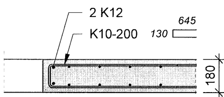
J3 Sérimynd 1 : 20
