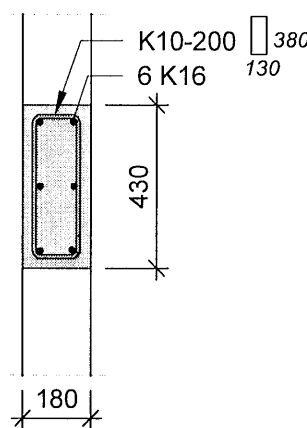
S3 1 : 20
