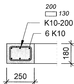
S4 1 : 20
