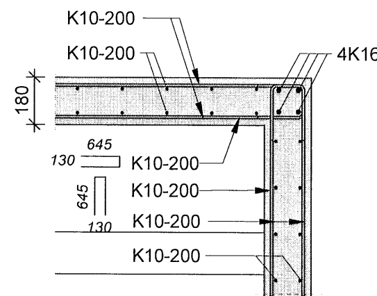
J4 Sérimynd 1 : 20
