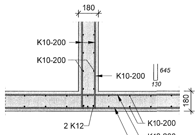
J2 Sérimynd 1 : 20
