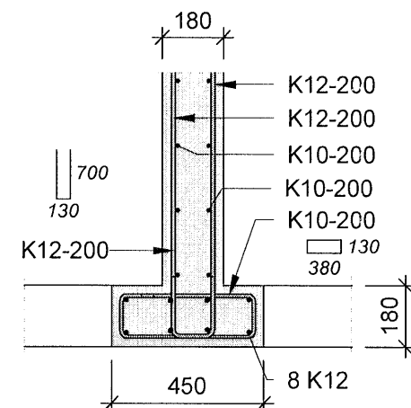
S5 1 : 20
