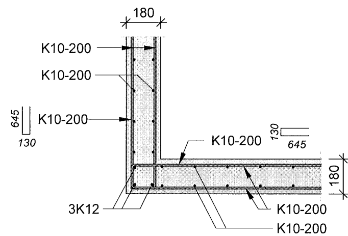
J1 Sérimynd 1 : 20
