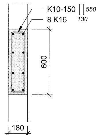
S2 1 : 20
