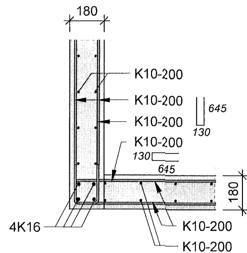
J5 Sérimynd 1 : 20
