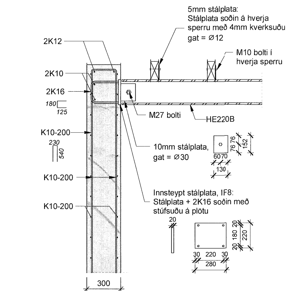
C38 Snið 1 : 20
