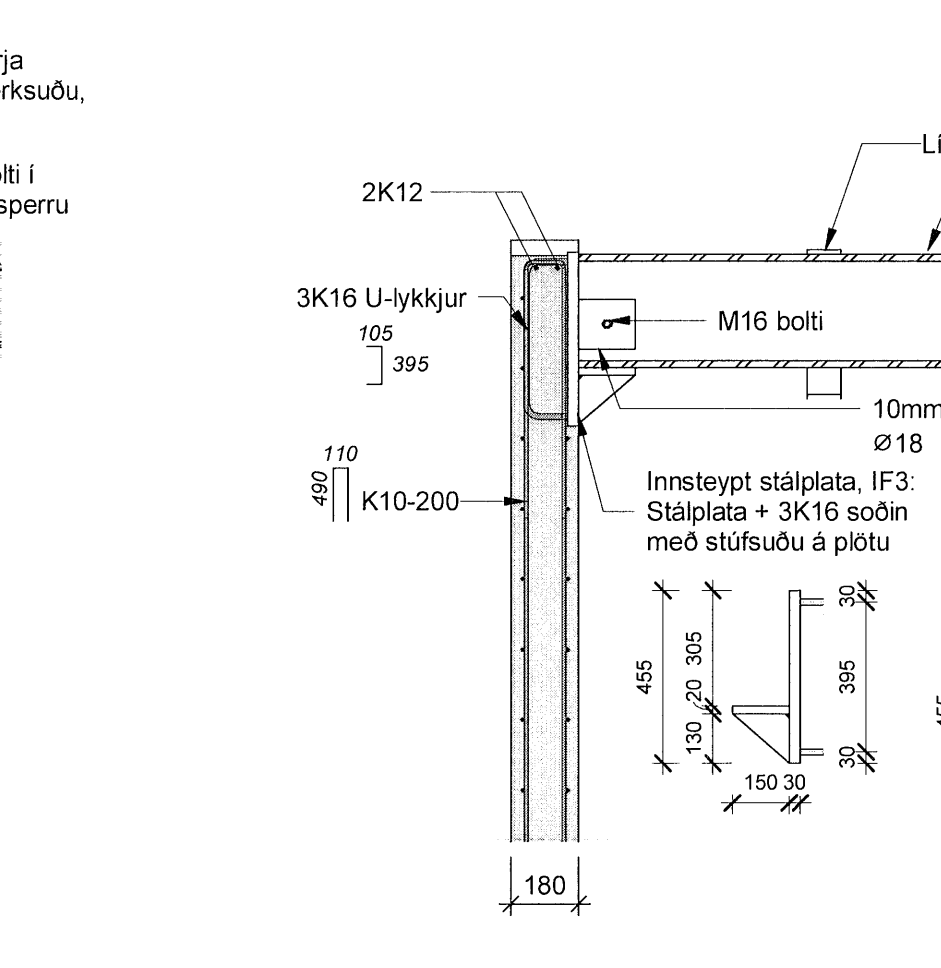
C39 Snið 1 : 20
