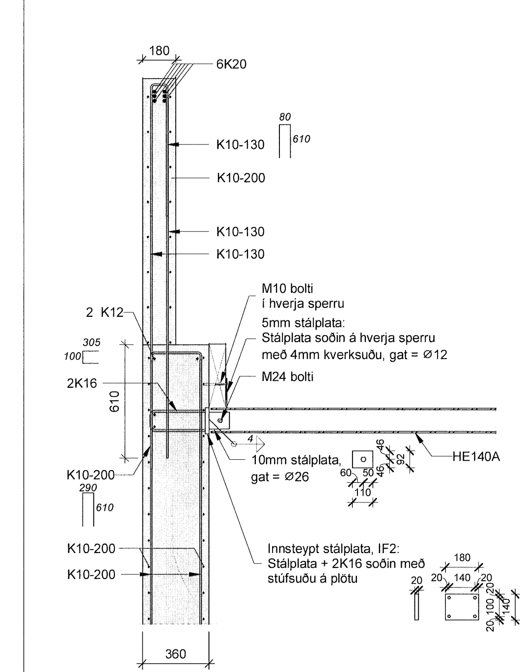
C37 Snið 1 : 20
