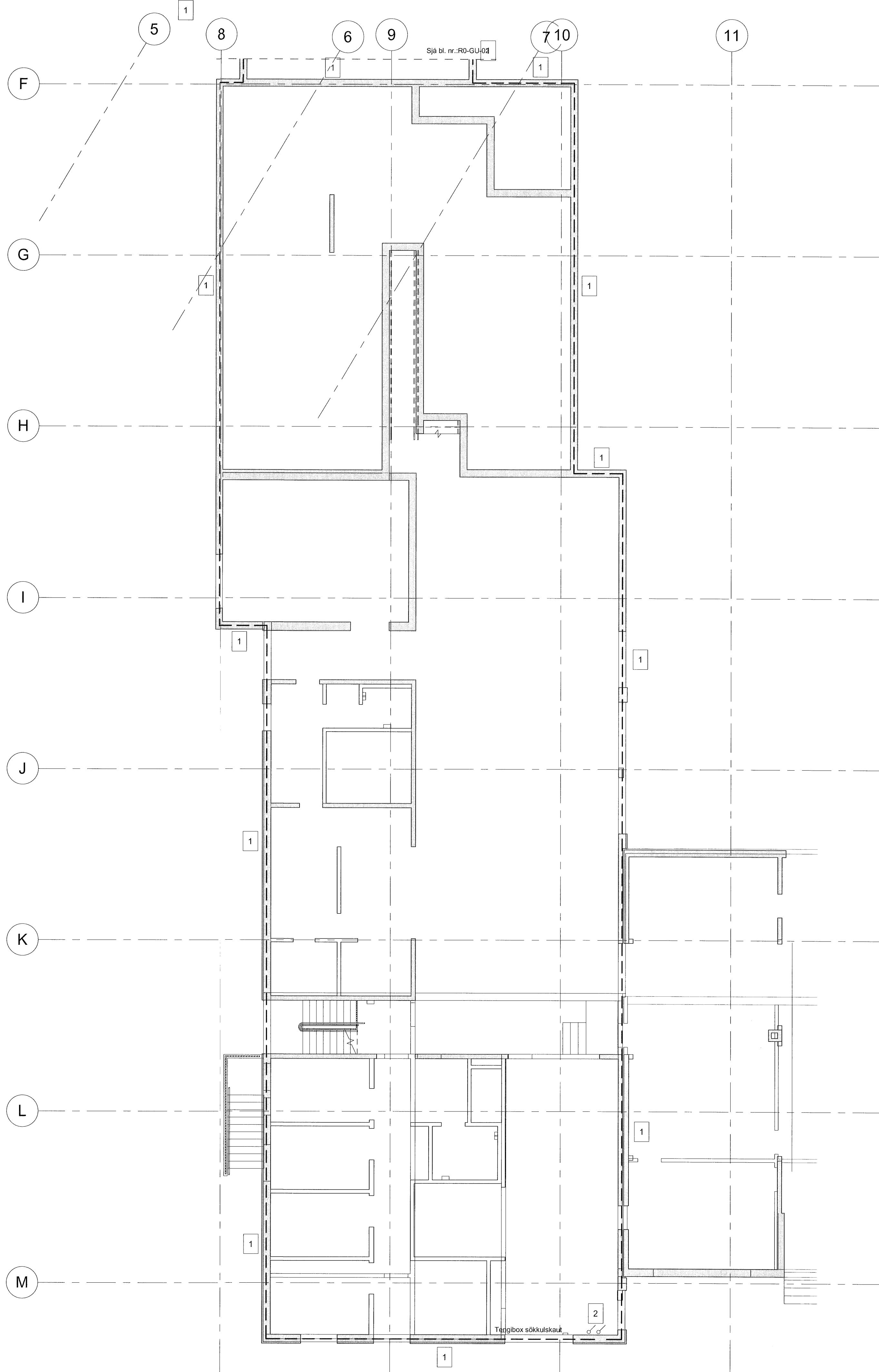
Sökkulskaut - 1. hluti
