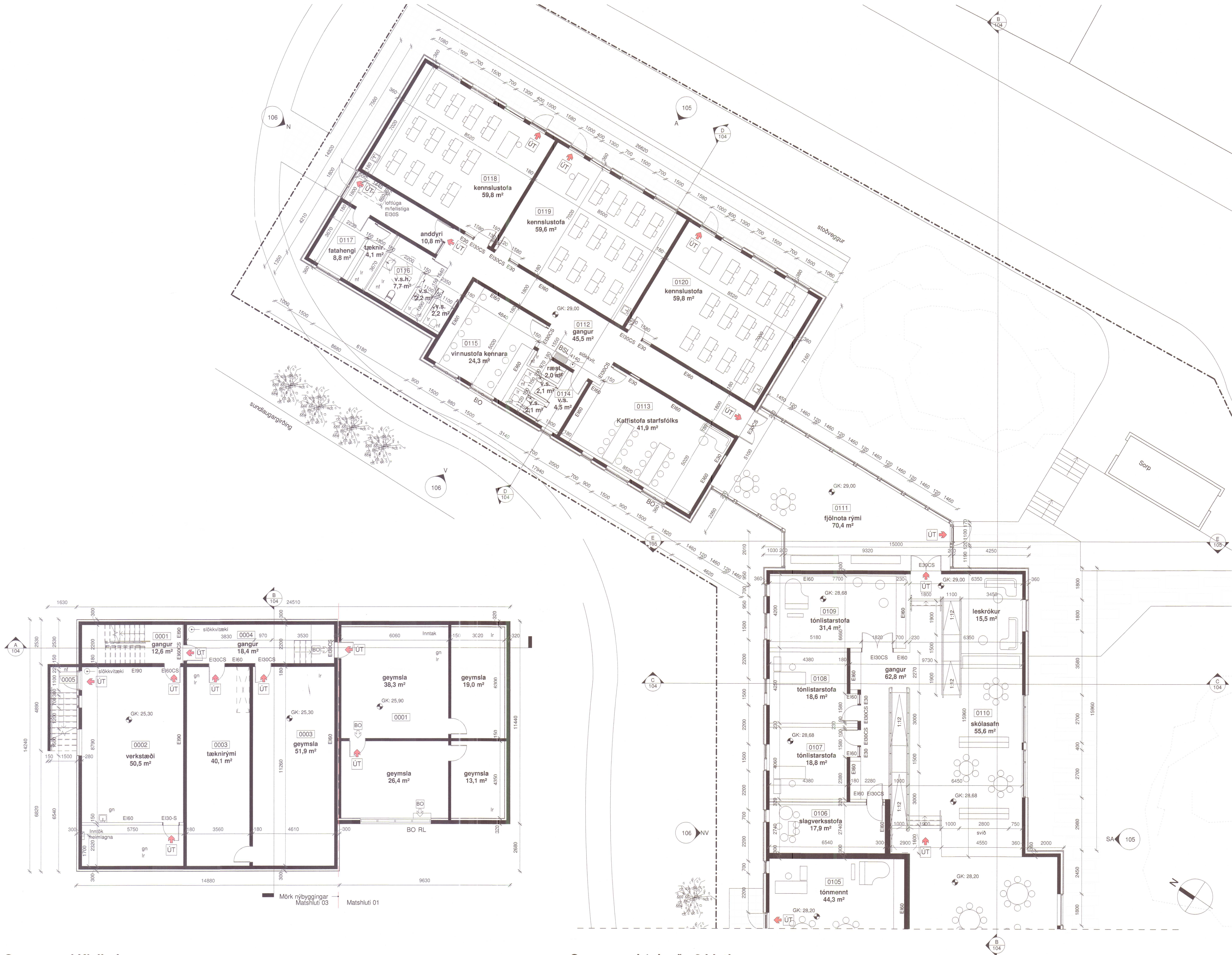
Grunnmynd Kjallari 1 : 100
