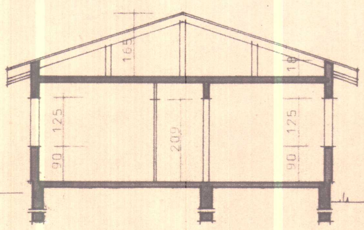
Skurður a-a
