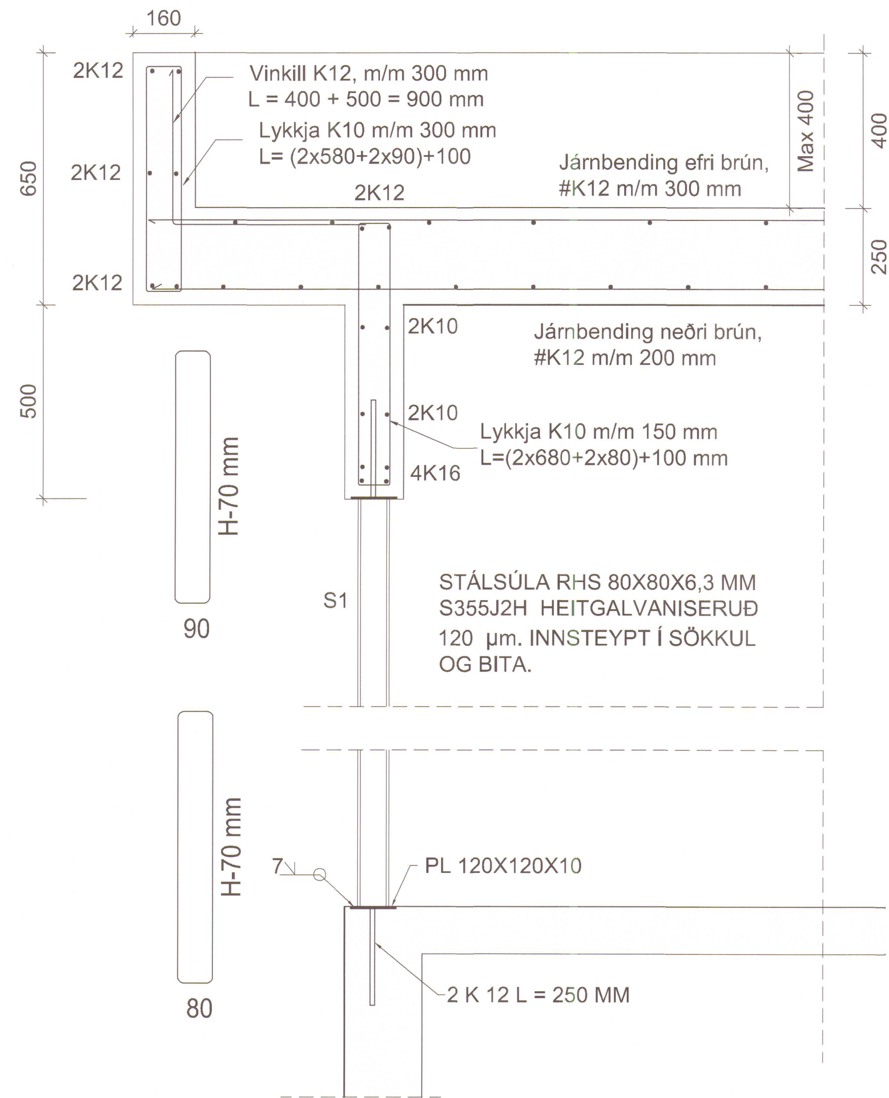
C Snið við stofuglugga 1:20
