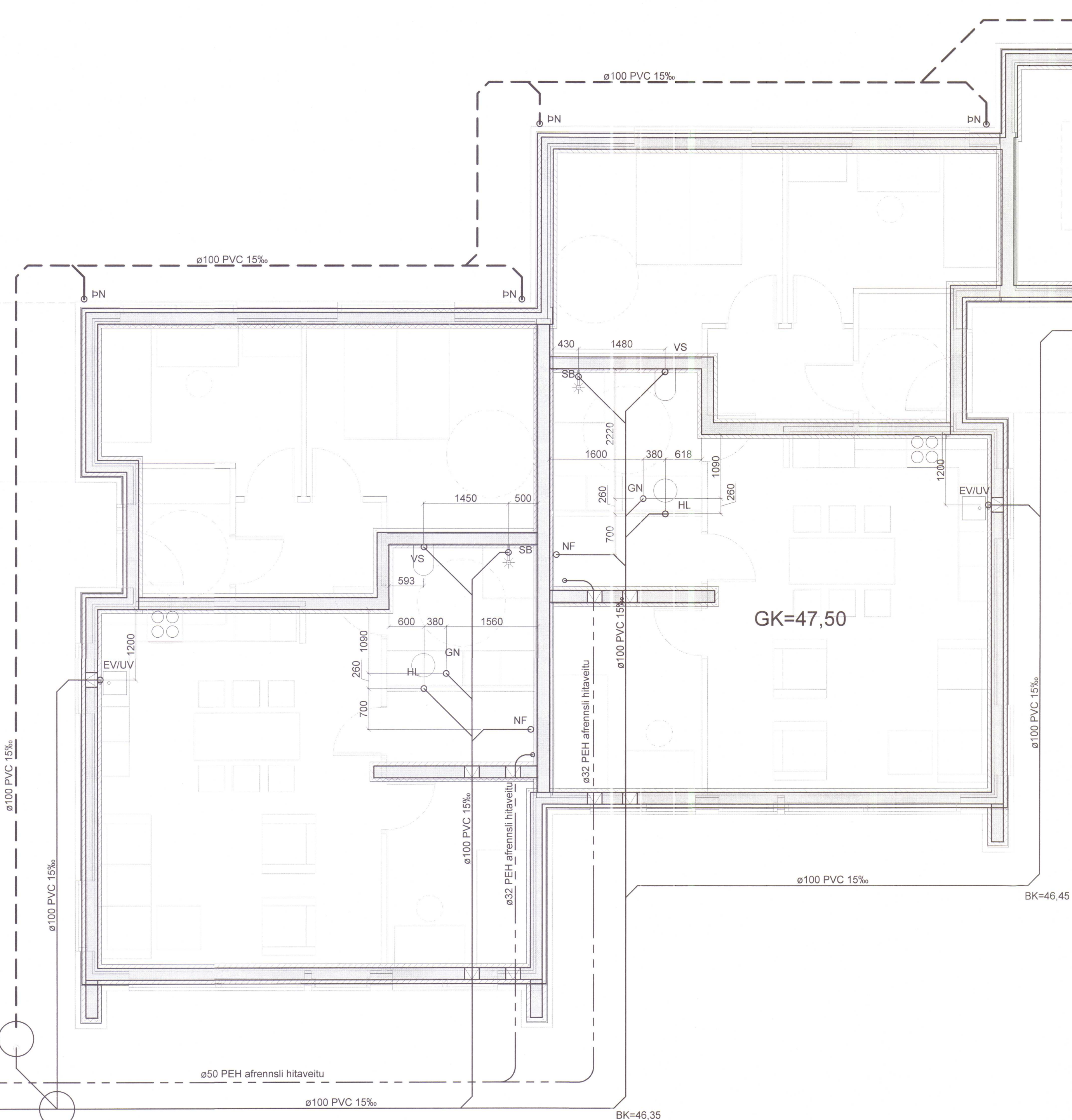
Frágangur jarðvatnslagna úr PVC 1:20
