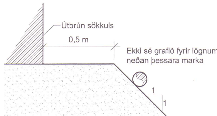
Lega lagna við hús 1:20
