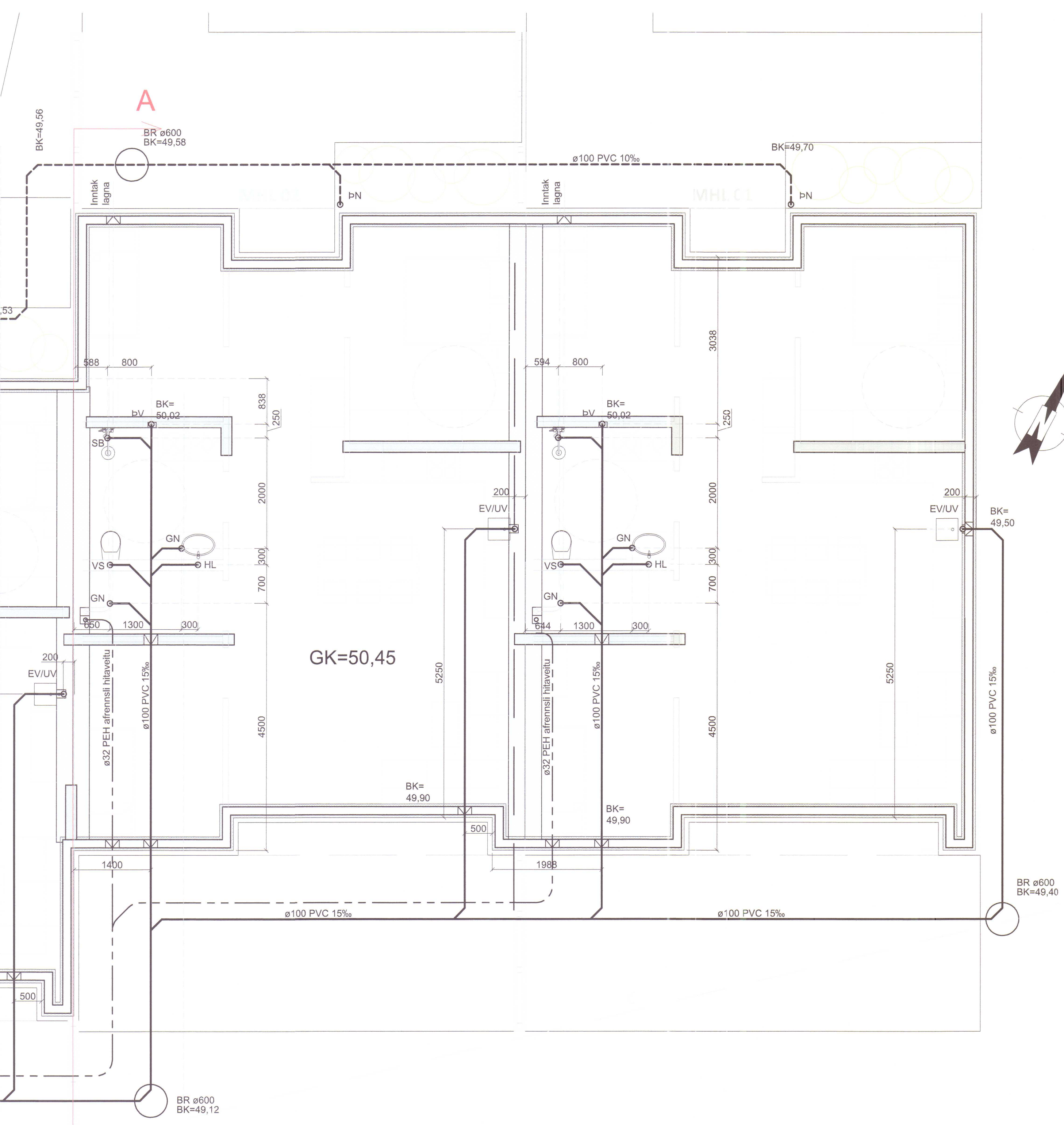
Grunnmynd Mkv. 1:50
