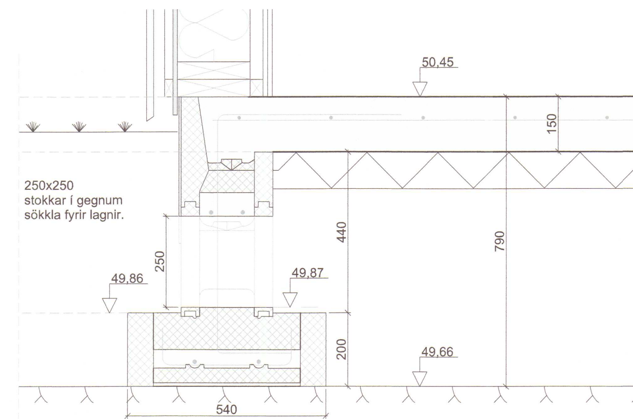
Stokkar fyrir lagnir í gegnum sökkla Mkv. 1:10
