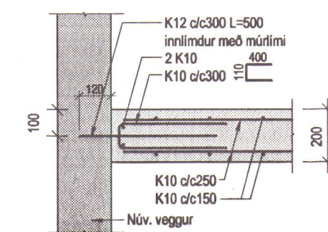
Snið F mk. 1:20
