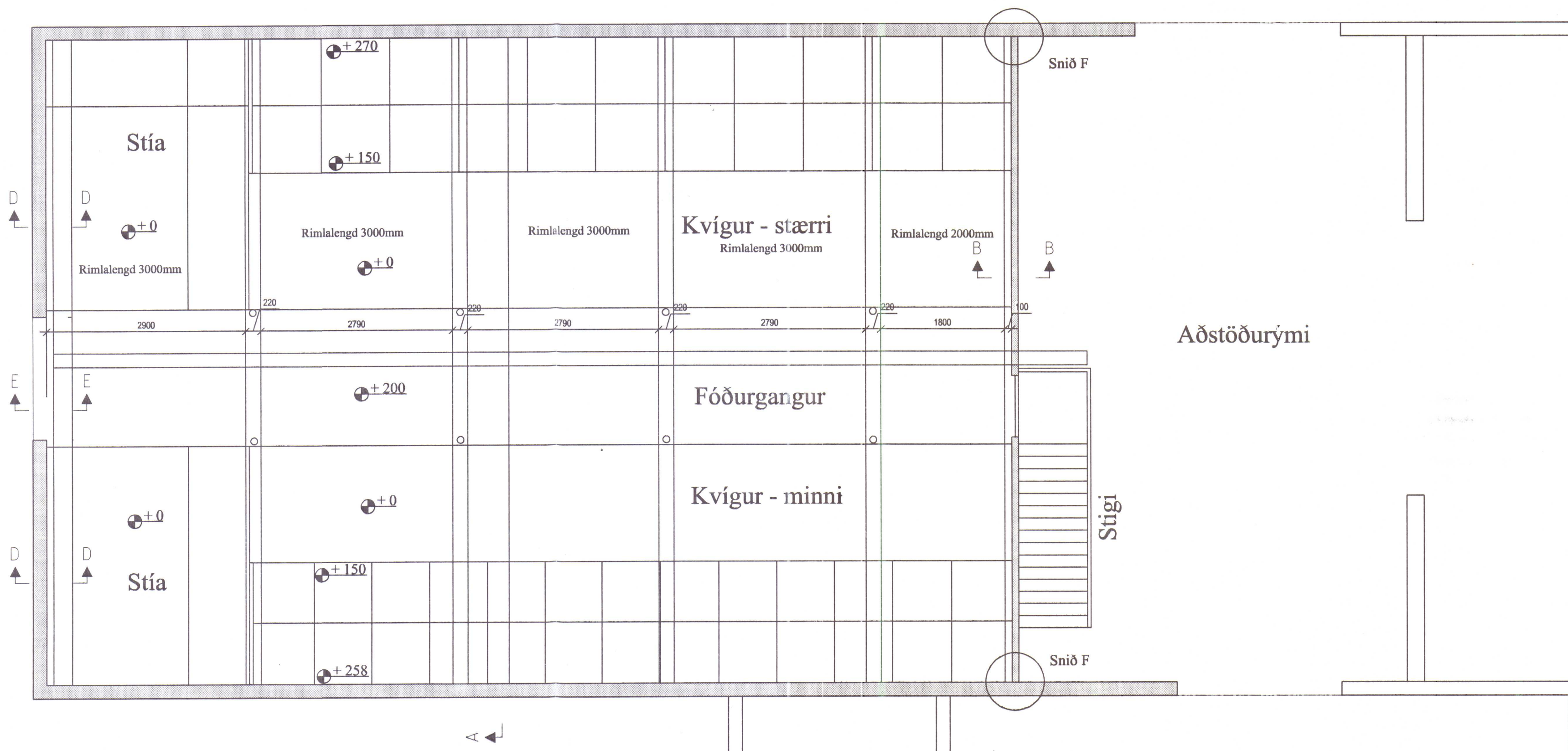
Grunnmynd kjallara mk. 1:50
