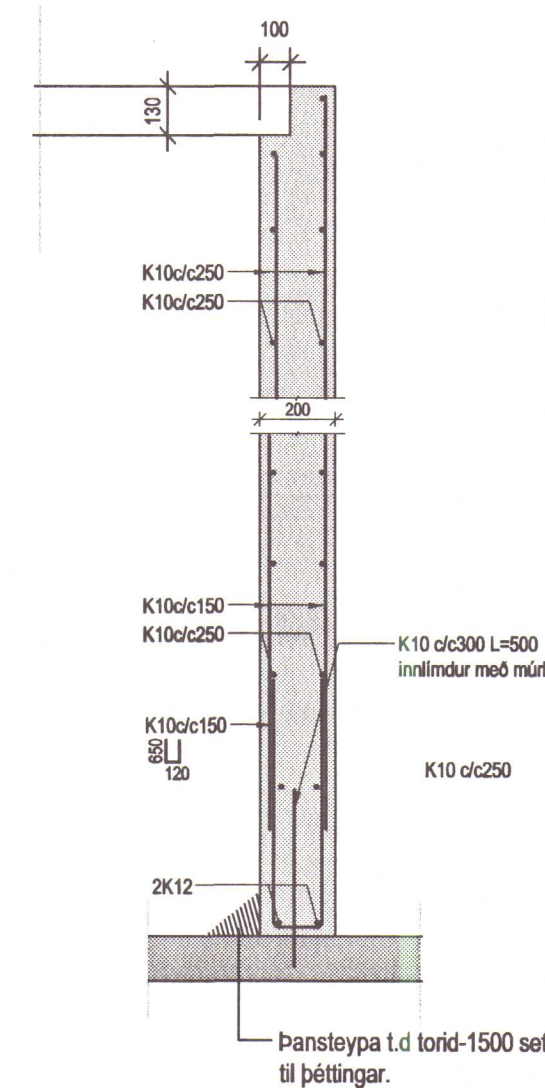
Snið B mk. 1:20
