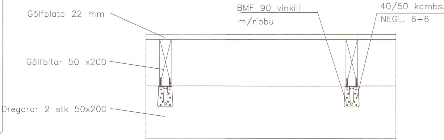
Festing dregarar/gólfbitar 1:10
