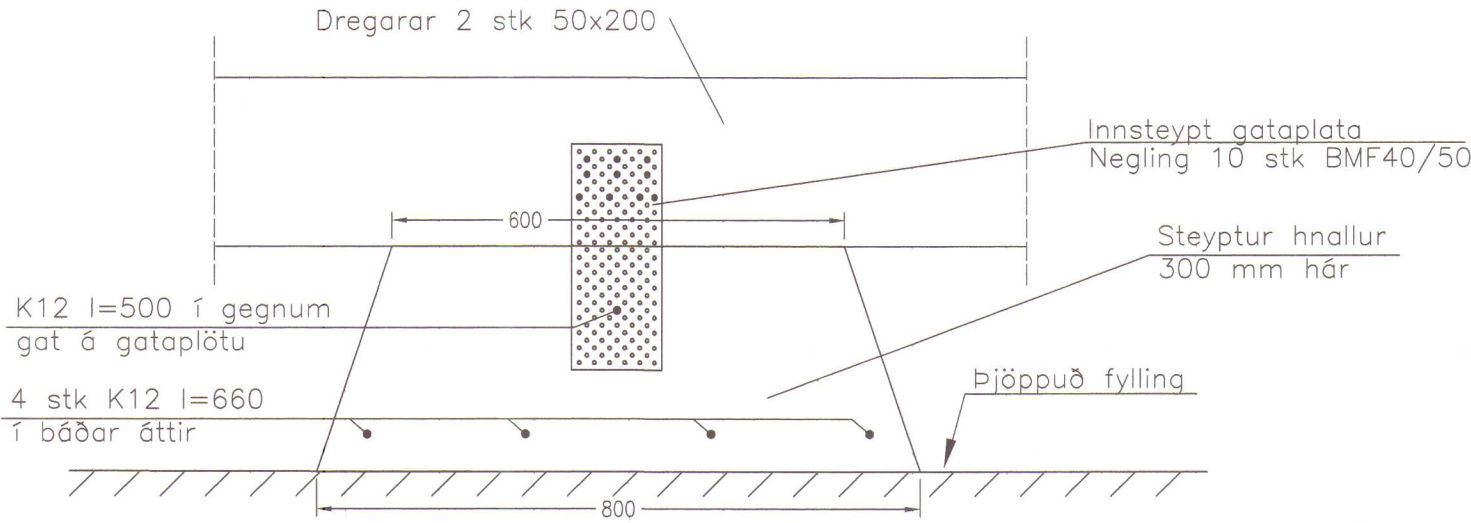
Snið B-B 1:10
