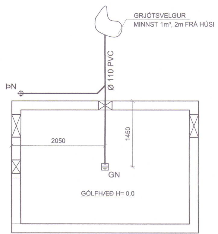
SÖKKULL, LAGNIR - GRUNNMYND mkv. 1:50
