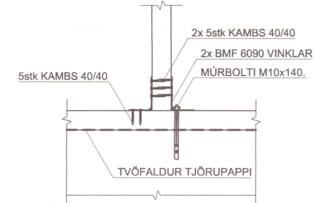
DEILI 2 mkv. 1:10
