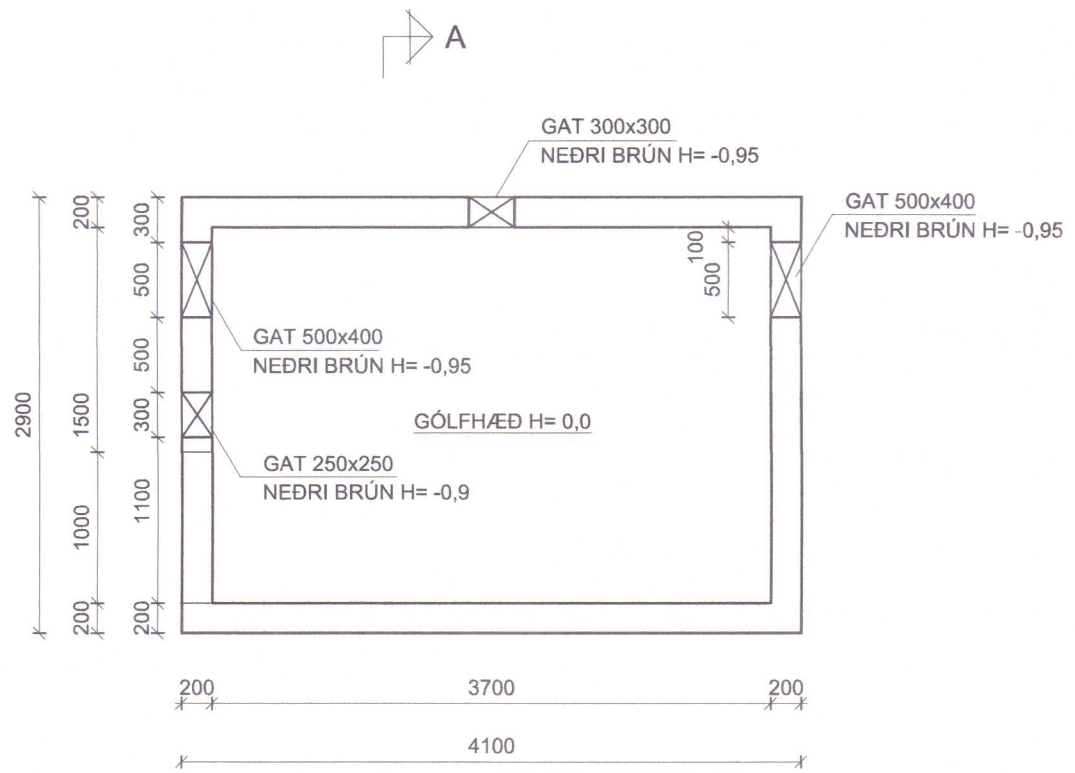
SÖKKULL - GRUNNMYND mkv. 1:50
