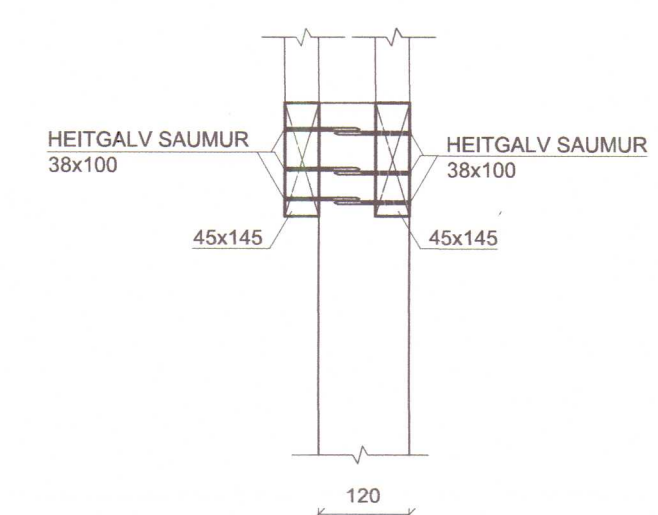
SNID C mkv. 1:10
