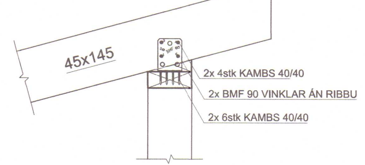
DEILI 4 mkv. 1:10
