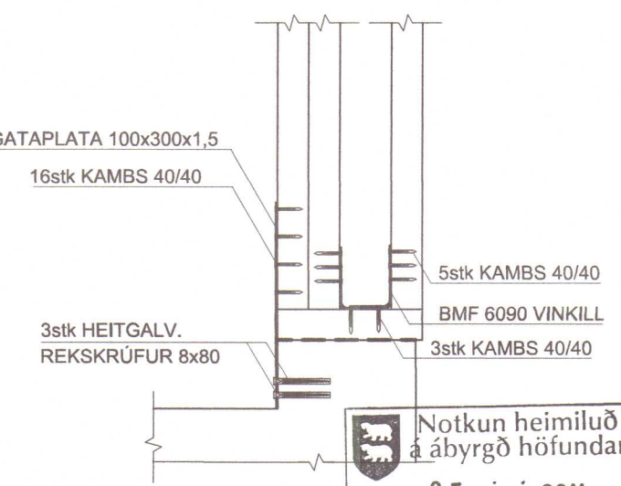
DEILI 4 mkv. 1:10
