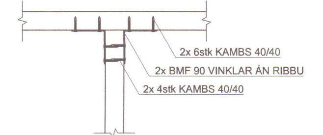
DEILI 1 mkv. 1:10
