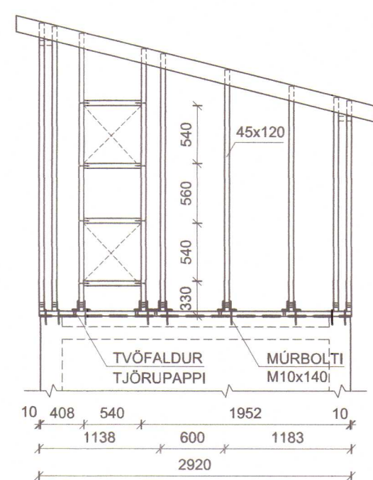
NORÐURVEGGUR mkv. 1:50
