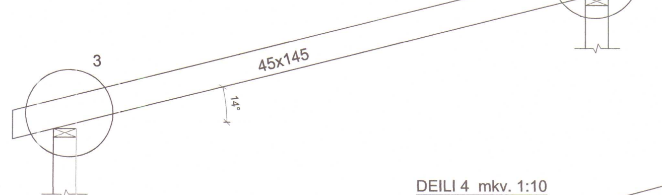
SNID D mkv. 1:20
