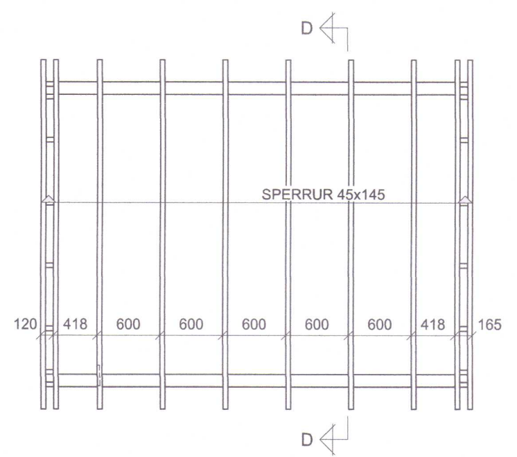
ÞAK - GRUNNMYND mkv. 1:50
