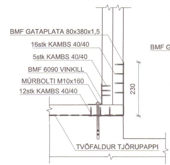
DEILI 3 mkv. 1:10
