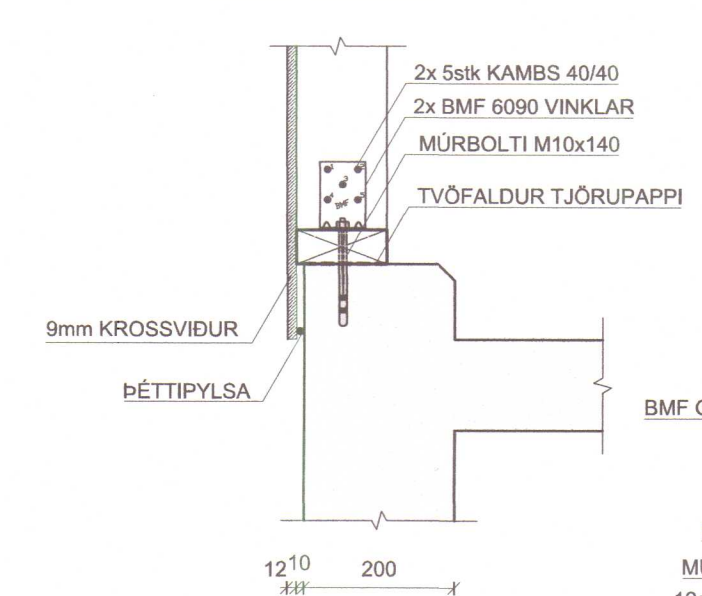
SNID B mkv. 1:10
