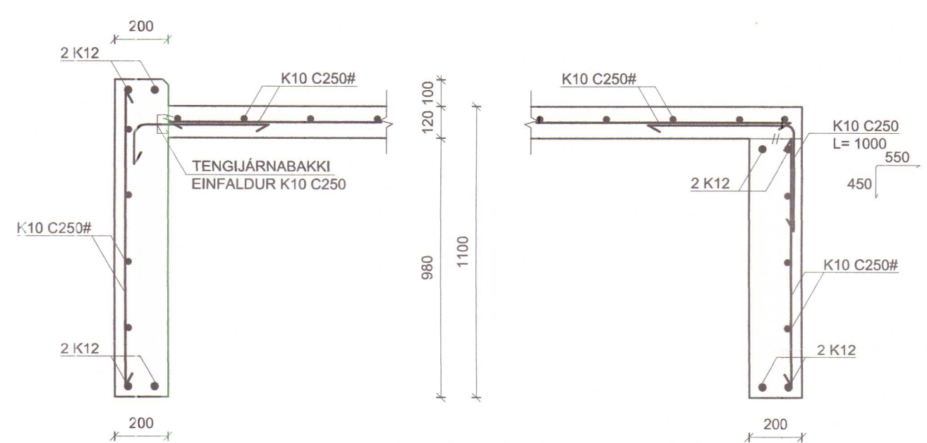
SNID A mkv. 1:20
