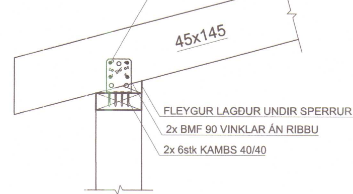
DEILI 3 mkv. 1:10
