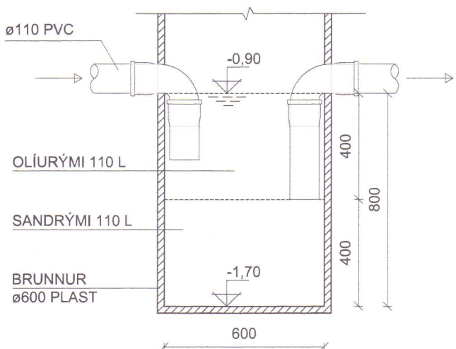
SAND- OG OLIUSKILJA A mkv. 1:20
