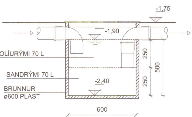
SAND- OG OLIUSKILJA B mkv. 1:20
