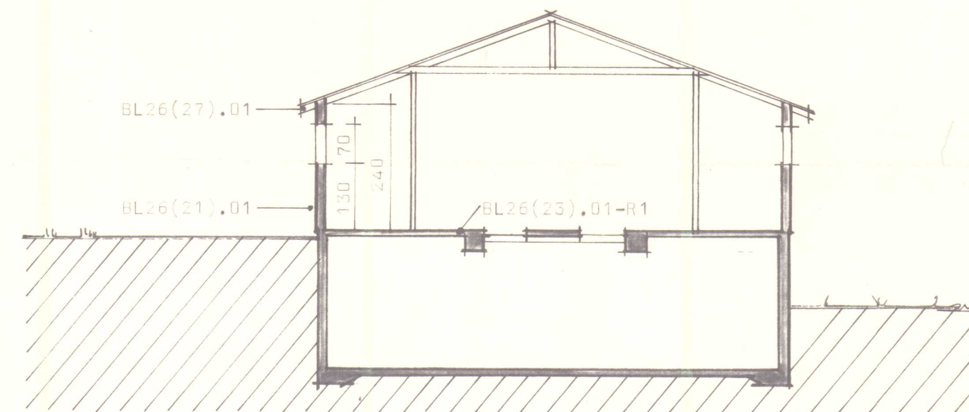
Þverskurður A-A
