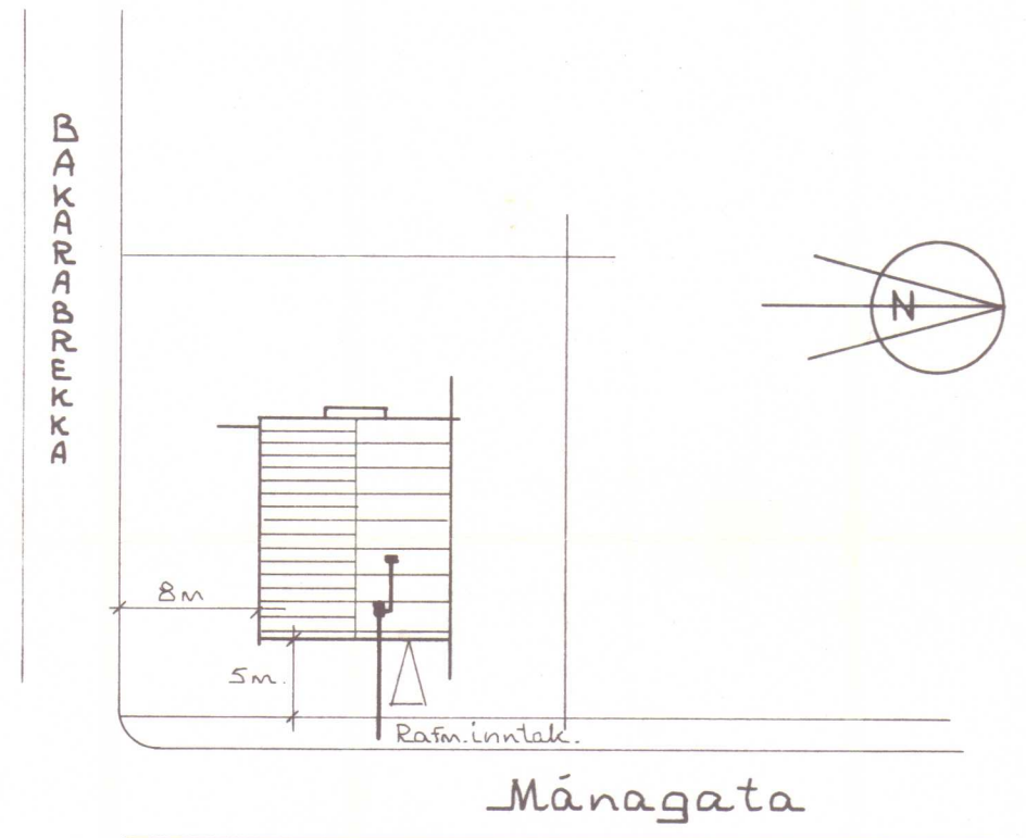
Afstöðumynd M=1:500
