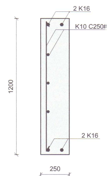
SNID A mkv. 1:20
