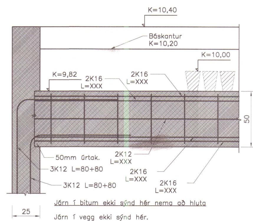
Snið 1 tengingu bita og veggja 1:20 Þringsnið
