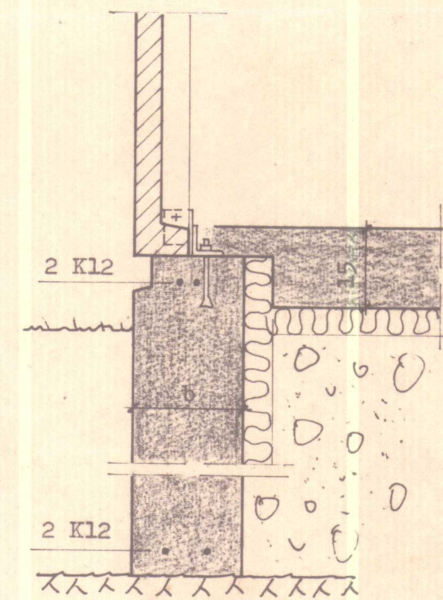
SNID Í SÖKKUL M. 1:10
