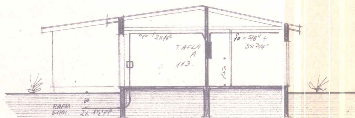
SNEIÐING A-A M 1:100
