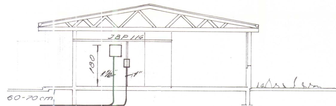
Skurður M. 1:100
