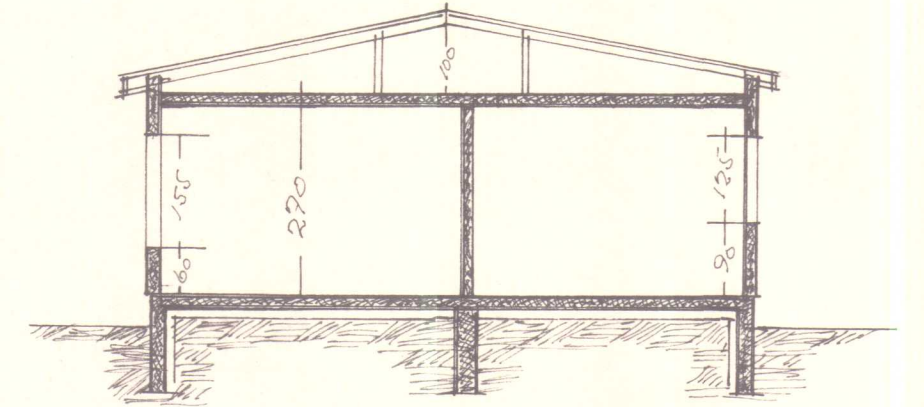
SKURÐUR A-A.
