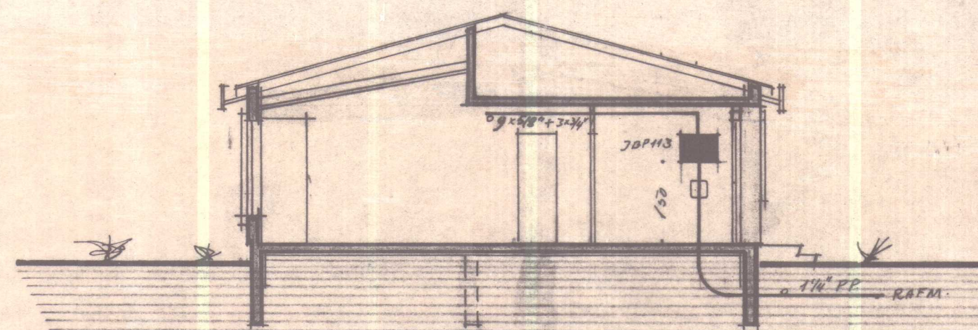
SNEIJING A-A M 1:100
