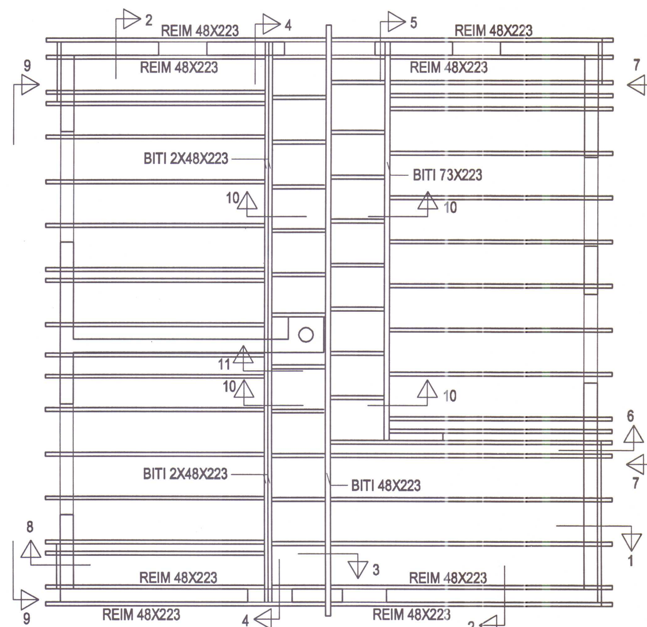
GRUNNMYND ÞAKVIÐA MKV. 1:50
