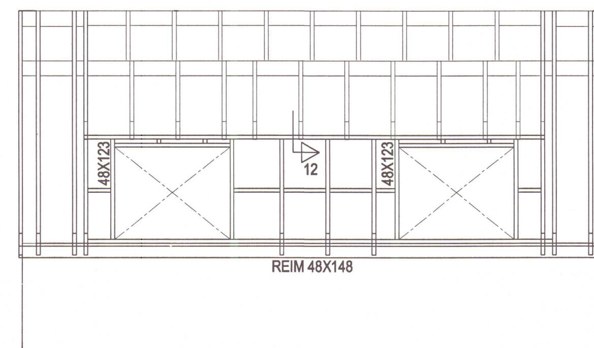
SNID 9-9 MKV. 1:50
