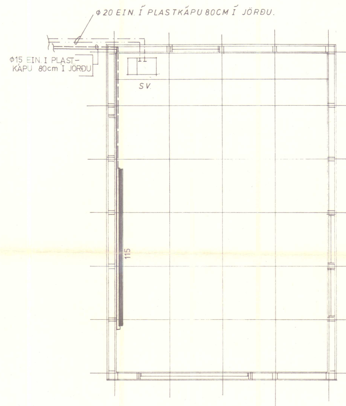
SNID B-B 1:10
