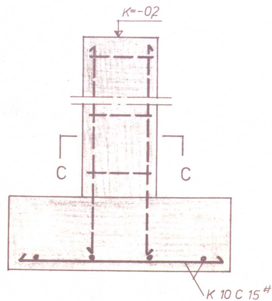
SNID B-B 1:10
