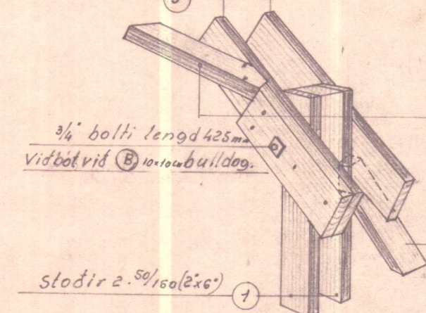
Sperra 2 150/200 (2x8") ③
