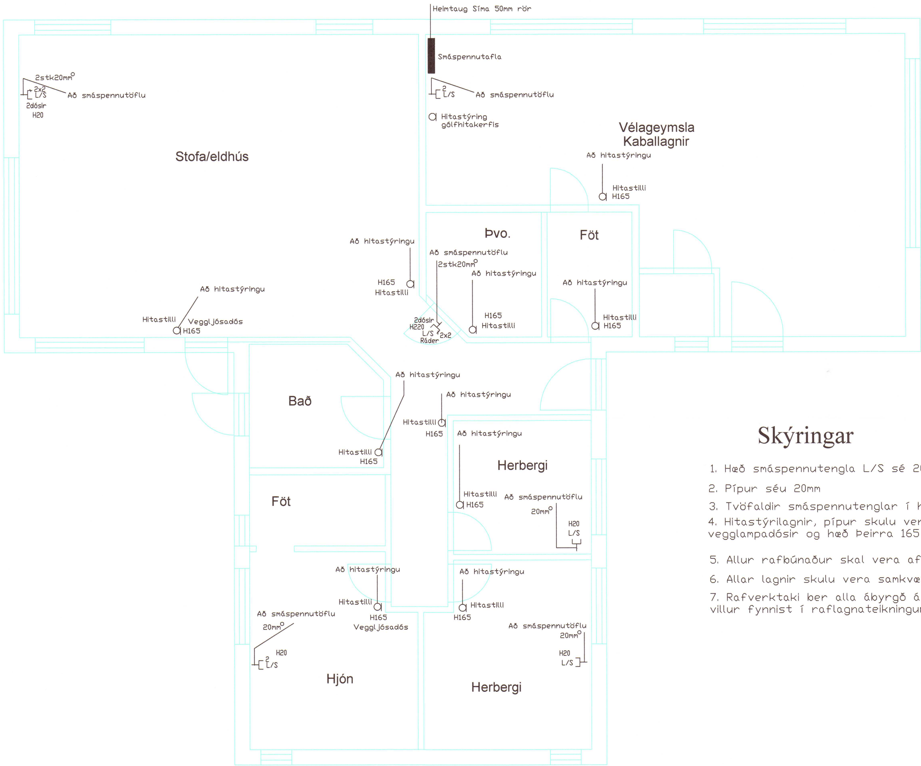
Grunnmynd M:1:50 Smáspenna
