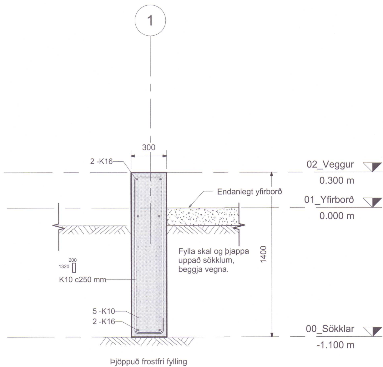
1 Snið gaflvegg 1 : 20
