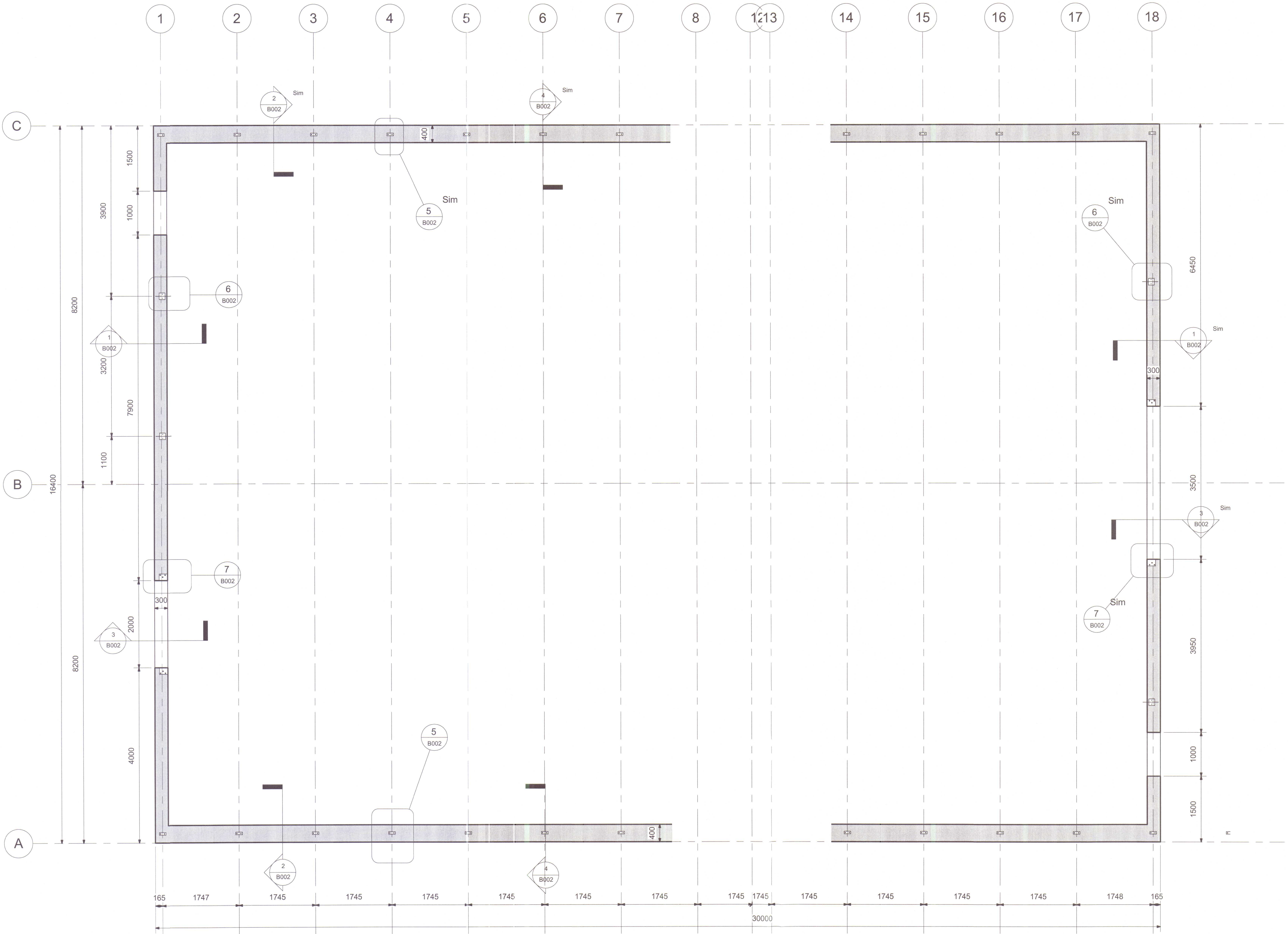
1 Botnplata, grunnmynd 1 : 50
