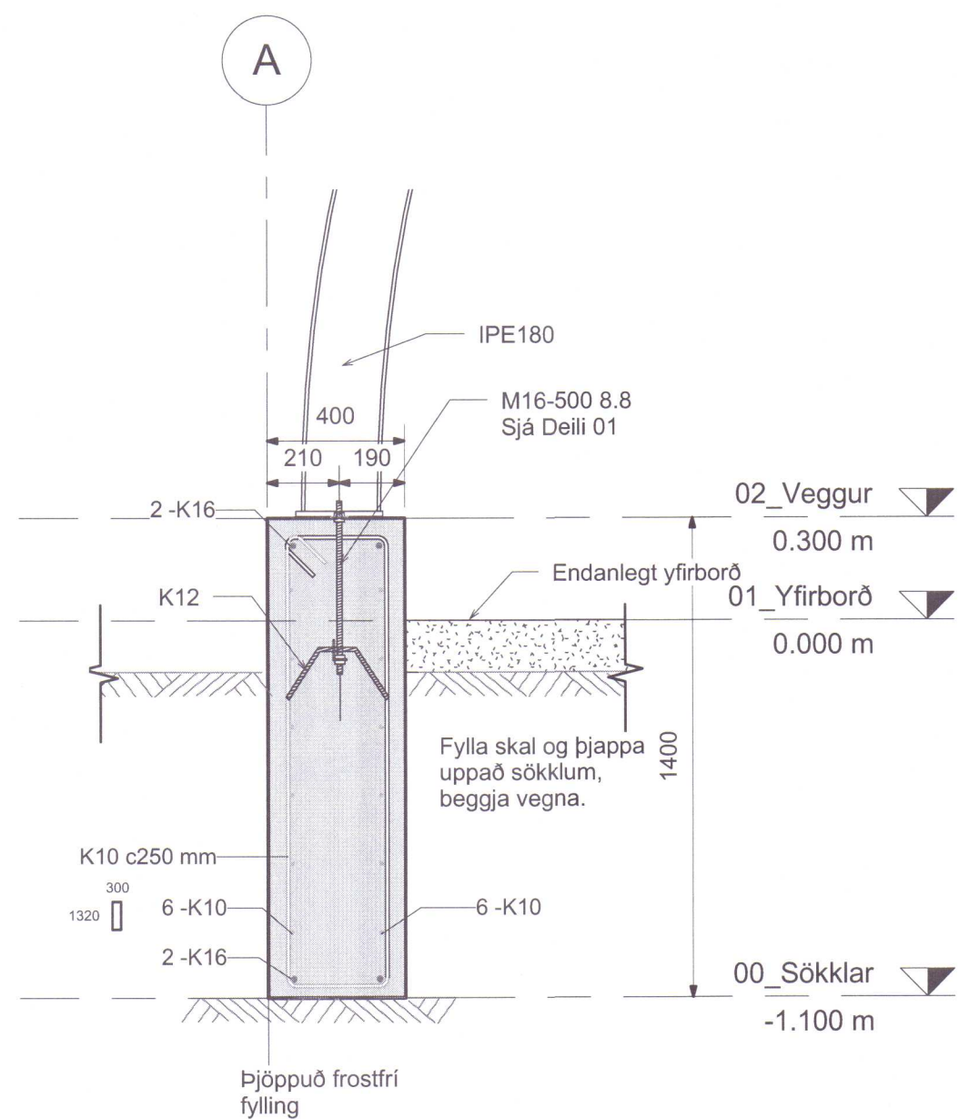
4 Snið festing 1 : 20
