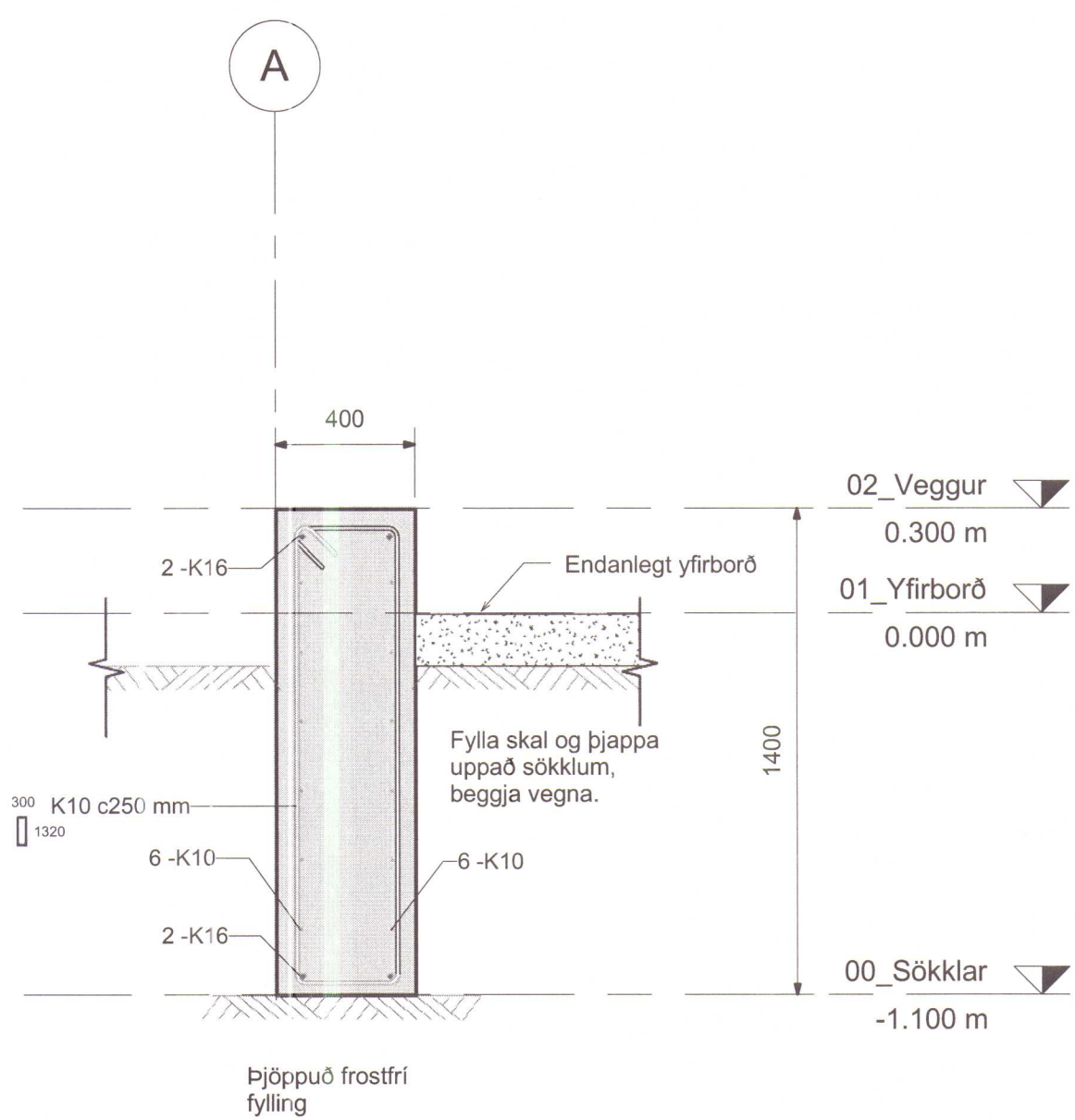
2 Snið langvegg 1 : 20
