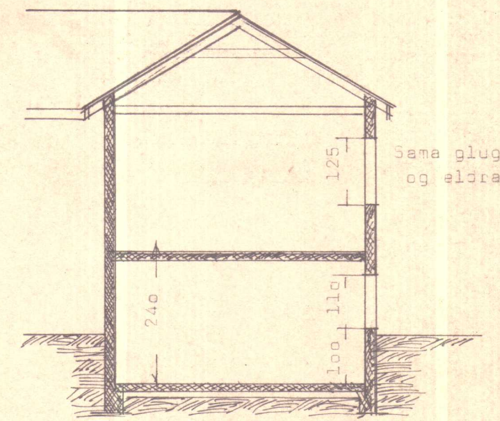
Skurður.
