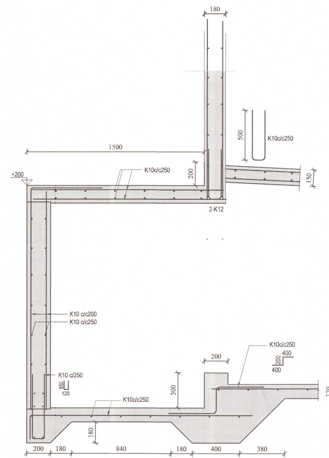
SNÍÐ A- MK. 1:20
