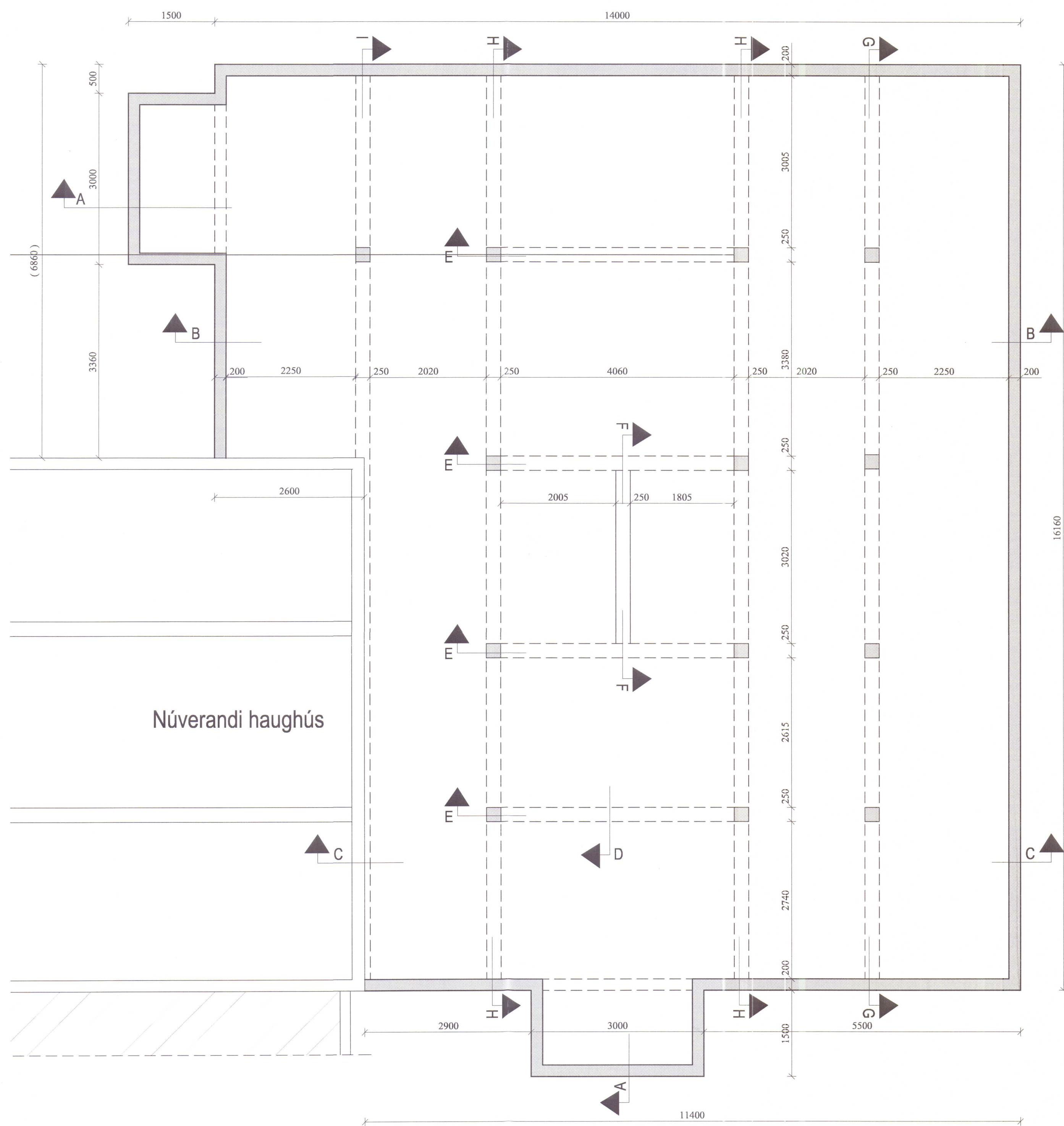
GRUNNMYND KJALLARA - MK. 1:50
