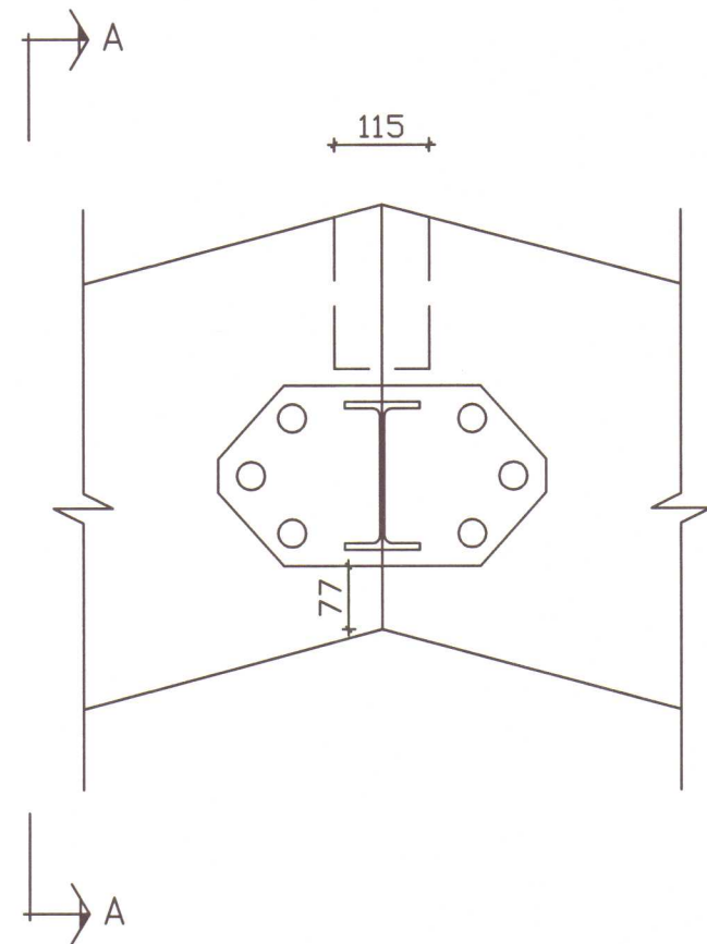
SAMSETNING A MK. 1:10
