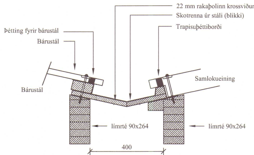
FRÁGANGUR Á SKOTRENNU VIÐ ELDRA HÚS . TILLAGA 1. MK. 1:10
