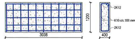
UNDIRSTAÐA, MKV. 1:50
